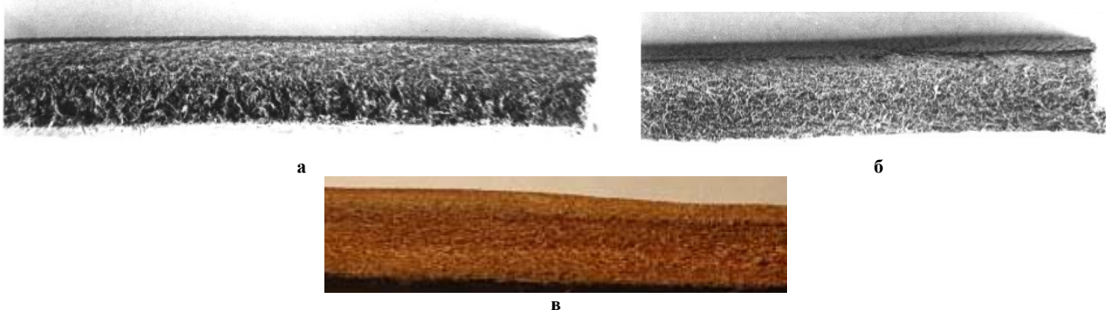
Рис. 8. Зразки поверхні торців деталі низу взуття з натуральної шкіри при вирубуванні: а - на пресі ПВГ-8-2-0; б - на пресовому обладнанні з ЛЕМД; в-б - на пресовому обладнанні з ЛЕМД з електромагнітним ПУЯ
