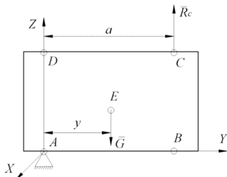
Рис. 2. Визначення положення центра ваги рівноваги має вигляд:
