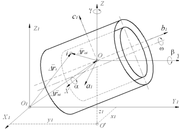
Рис. 4. До математичної моделі руху системи бак-барaban
