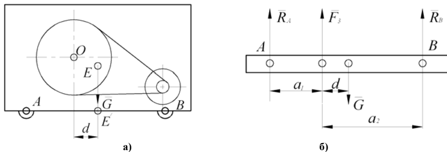
Рис. 3. Визначення положення центра ваги G – вага машини; F_3 – збурююча (відцентрова) сила; AB – днище машини; точки A і B – місця кріплення опорних катків на днищі
