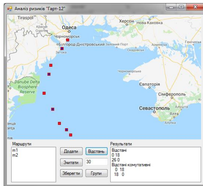
Рис. 4. Розрахунок метрик R(M_1, M_2) і R(M_2, M_1)
