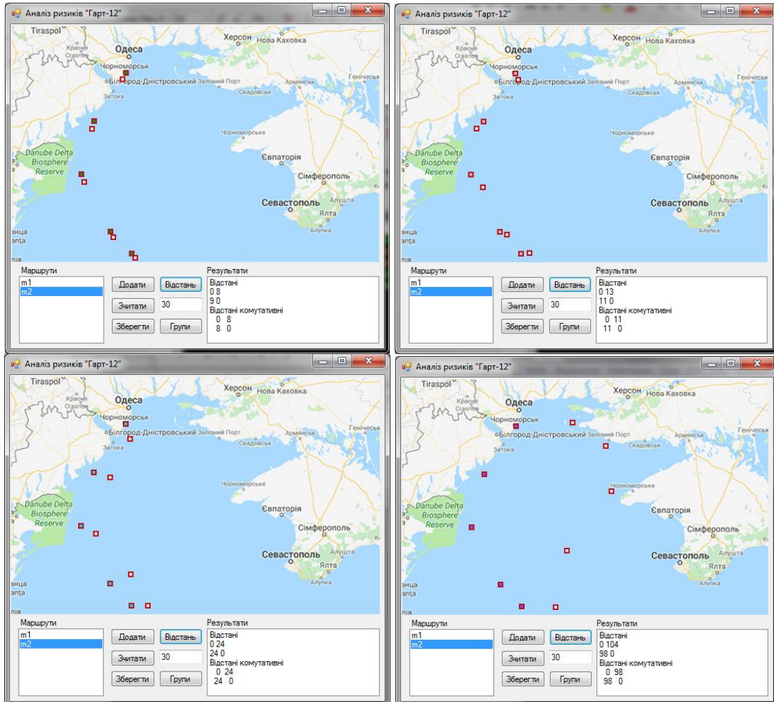
Рис. 5. Приклади обчислення метрики (7)
