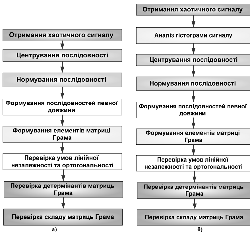
Рис 2. Послідовність (а) та доповнена послідовність (б) методу визначення оптимального з точки зору апаратних витрат базису хаос-підносійних.
