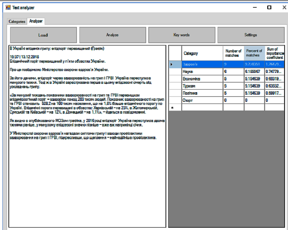
Рис. 5. Інтерфейс системи тематичного сортування новин
