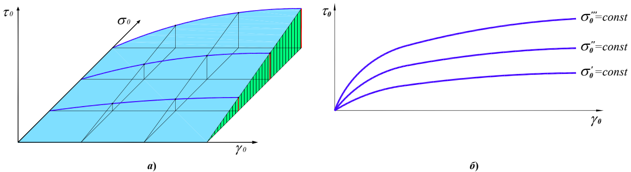
Рис. 2. Графічна інтерпретація залежностей А.І. Боткіна а) поверхня деформування б) зрізи поверхні площинами \sigma_0 = const
