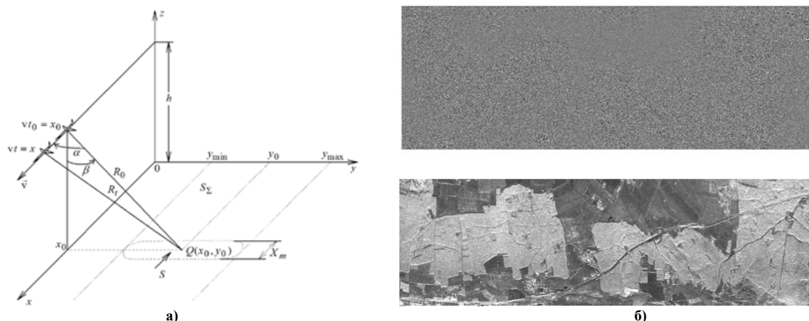
Рис. 1. Загальна схема синтезу апертури (а) і приклад формування радіолокаційного зображення до і після синтезу (б)
