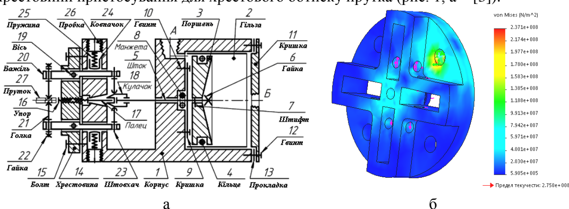
Рисунок 1 – Пристосування для хрестового обтиску прутка (а), вузли напруження хрестовини von Mises (б)
