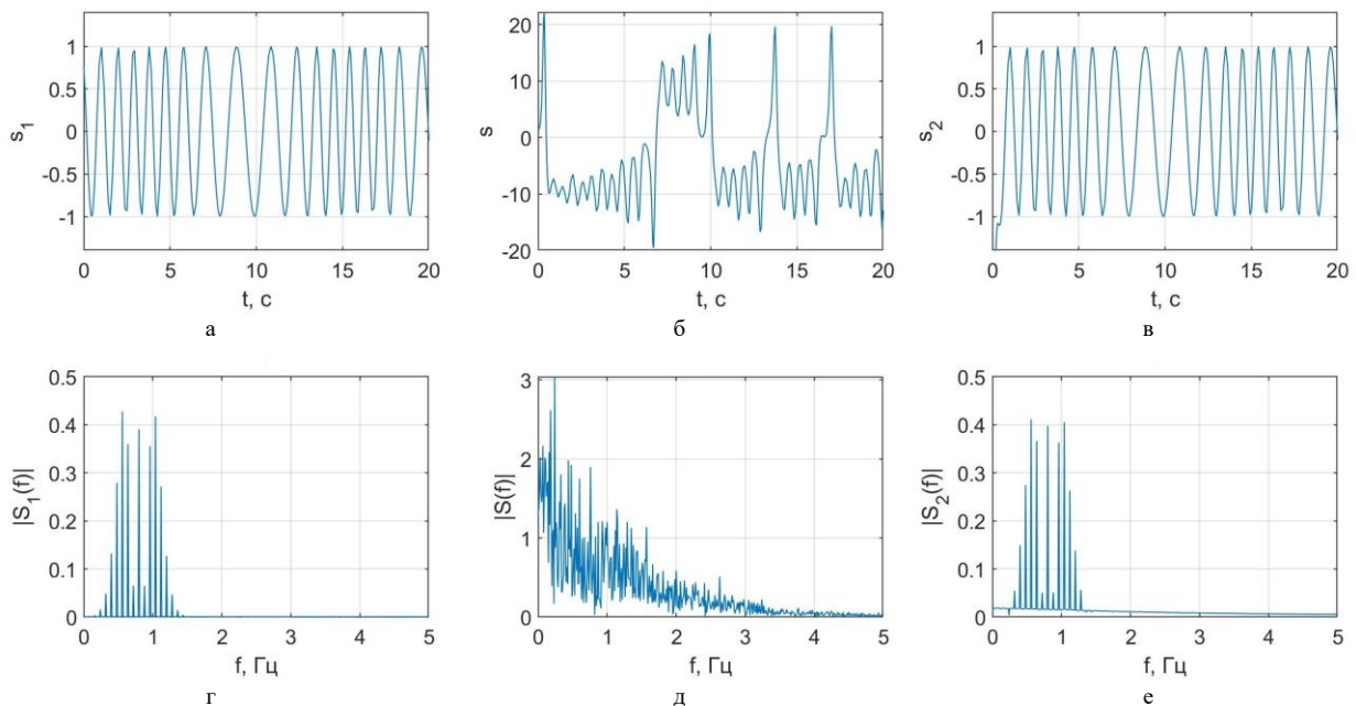
Рис. 7. Хаотичне маскування тестового вузькосмугового ЧМ-сигналу: сигнал на вході системи передачі та його амплітудний спектр – а), г); сигнал, переданий каналом зв'язку та його спектр – б), д); сигнал на виході приймальної системи та його спектр – в), е)
