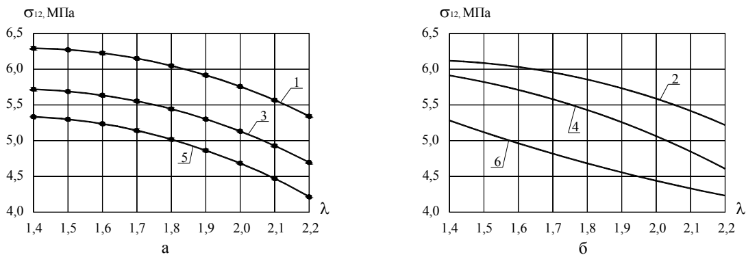
1, 2 – температура T = 80 \text{ }^{\circ}\text{C} ; 3, 4 – температура T = 110 \text{ }^{\circ}\text{C} ; 5, 6 – температура T = 140 \text{ }^{\circ}\text{C} Рис. 7. Залежності міцності на розрив поперек орієнтації структури зразка, виготовленого з полівінілхлориду, від ступеня витяжки: а – апроксимація експериментальних даних; б – аналітичні залежності
