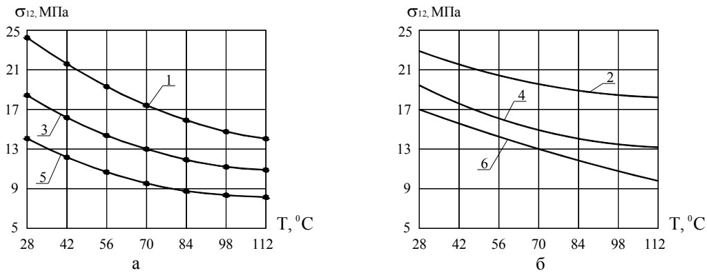
1, 2 – ступінь витяжки \lambda = 1 ; 3, 4 – ступінь витяжки \lambda = 2,5 ; 5, 6 – ступінь витяжки \lambda = 4,0 Рис. 4. Залежності міцності на розрив поперек орієнтації структури поліетиленового зразка від температури: а – апроксимація експериментальних даних; б – аналітичні залежності
