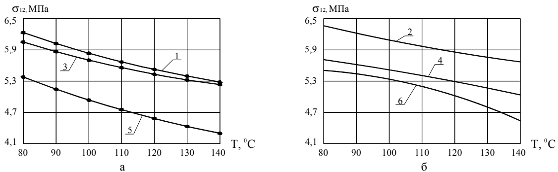
1, 2 – ступінь витяжки \lambda = 1 ; 3, 4 – ступінь витяжки \lambda = 1,6 ; 5, 6 – ступінь витяжки \lambda = 2,2 Рис. 6. Залежності міцності на розрив поперек орієнтації структури зразка, виготовленого з полівінілхлориду, від температури: а – апроксимація експериментальних даних; б – аналітичні залежності
