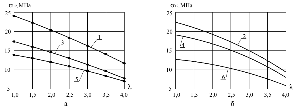
1, 2 – температура T = 28 \text{ }^{\circ}\text{C} ; 3, 4 – температура T = 70 \text{ }^{\circ}\text{C} ; 5, 6 – температура нагрівання T = 112 \text{ }^{\circ}\text{C} Рис. 5. Залежності міцності на розрив поперек орієнтації структури поліетиленового зразка від ступеня витяжки: а – апроксимація експериментальних даних; б – аналітичні залежності
