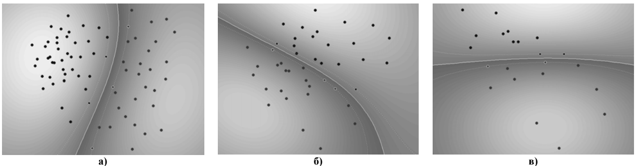
Рис. 6. Розміщення груп точок на площині та їх розділення гаусівським класифікатором
