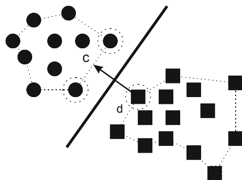
Рис. 2. Перший підхід класифікації
