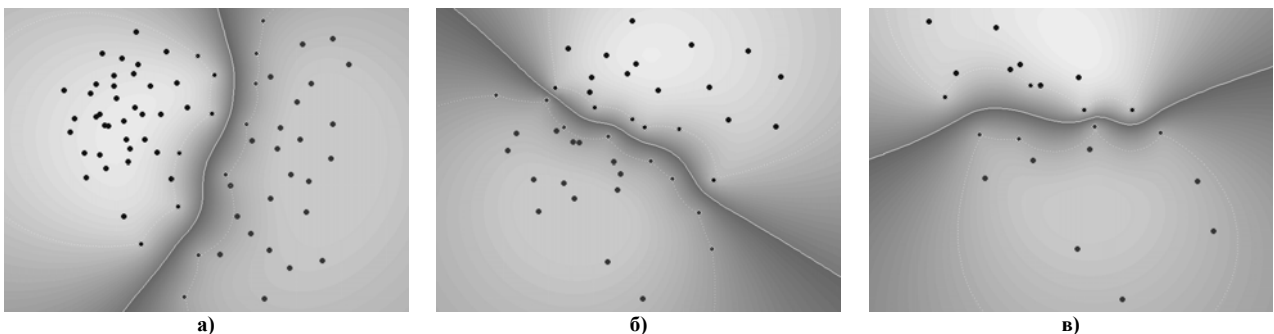
Рис. 7. Розміщення груп точок на площині і їх розділення експоненційним класифікатором:
