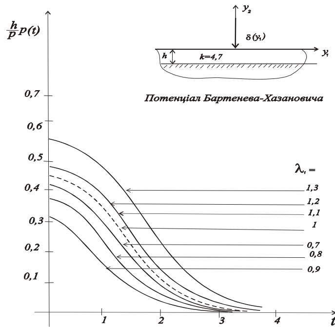
Рис. 2 – Контактна взаємодія під дією вертикальної сили у випадку потенціалу Бартенева-Хазановича
