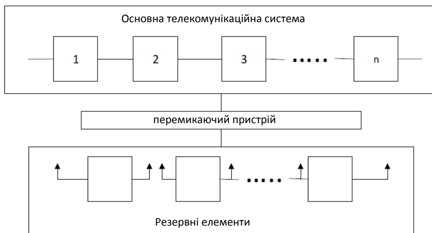
Рис. 3. Схема ковзаючого резервування
