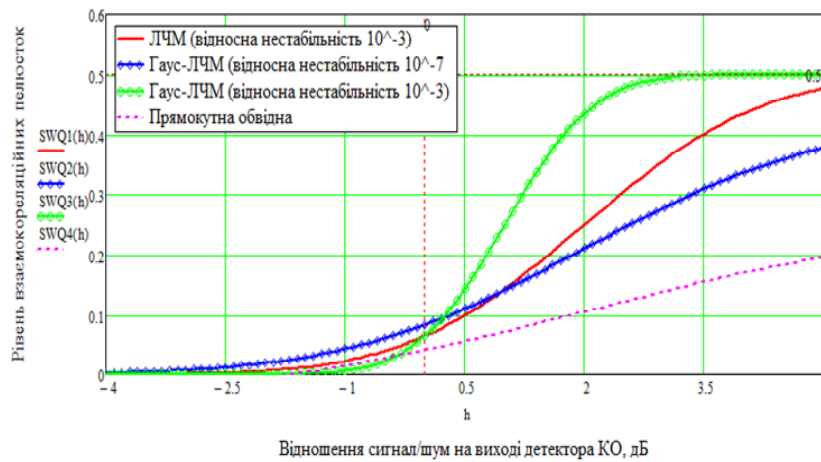
Рис. 6. Залежність нормованого рівня взаємкореляційних членів від відношення сигнал/шум на виході детектора комплексної обвідної
