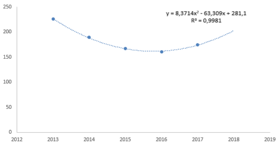
Рис. 2. Квадратична модель тренду надходження іноземних інвестицій за 2013–2017 рр.
