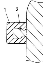
Рис. 3. Поясок шпулетримача виготовлений з полімеру: 1 – поясок з полімеру; 2 – металічний шпулетримач [18]
