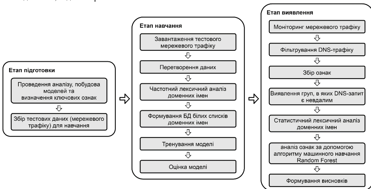
Рис. 2. Загальна схема функціонування методу виявлення бот-мереж, що використовують технологію «потік доменів»
