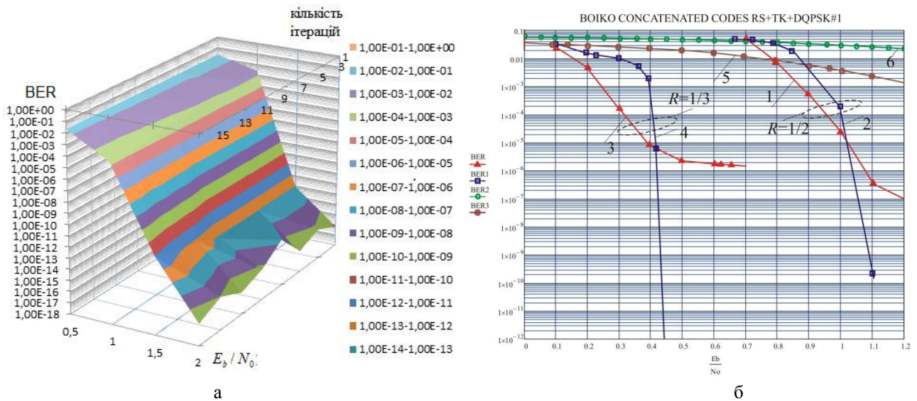
Рис. 3. Залежності завадостійкості для запропонованої каскадної СКК: PC (255, 239)+TK ( L=16384 бітів; 10 ітерацій)+DQPSK:
