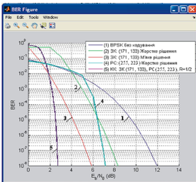
Рис. 2. Залежності ймовірності біткової помилки (BER) від відношення сигнал/шум ( E_b / N_0 )
