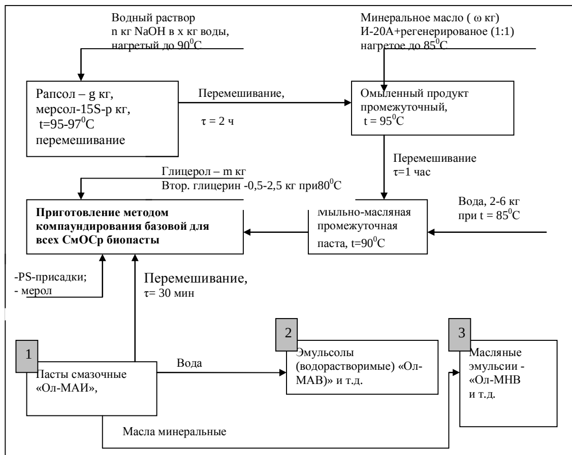
Рис.5. Структурно-логическая схема технологии производства базовой масляной биопасты эмульсолов и масляных эмульсий по рецептуре примера 2
