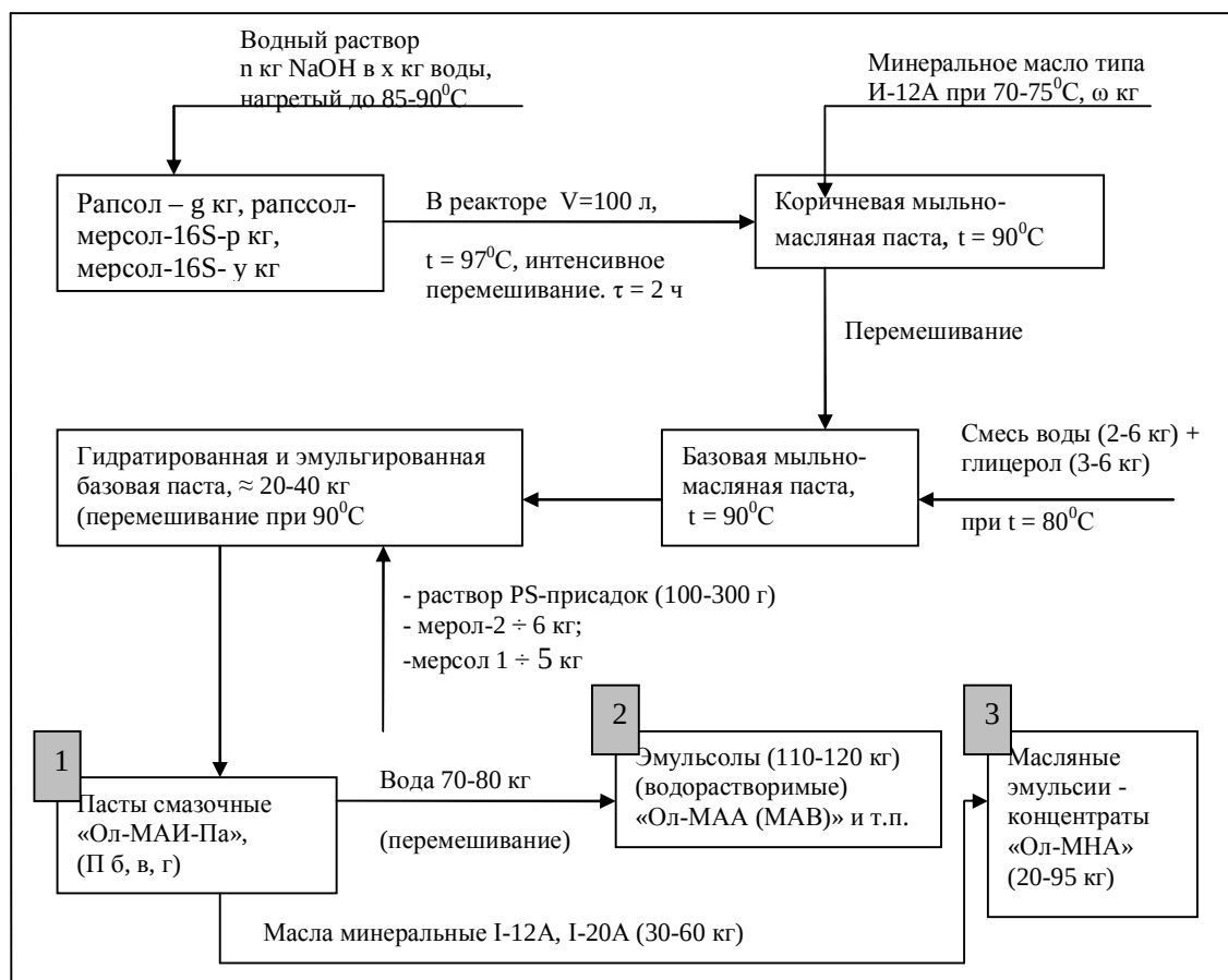
Рис. 4. Структурно-логическая схема производства базовой масляной биопасты эмульсолов и масляных эмульсий по рецептуре примера 1
