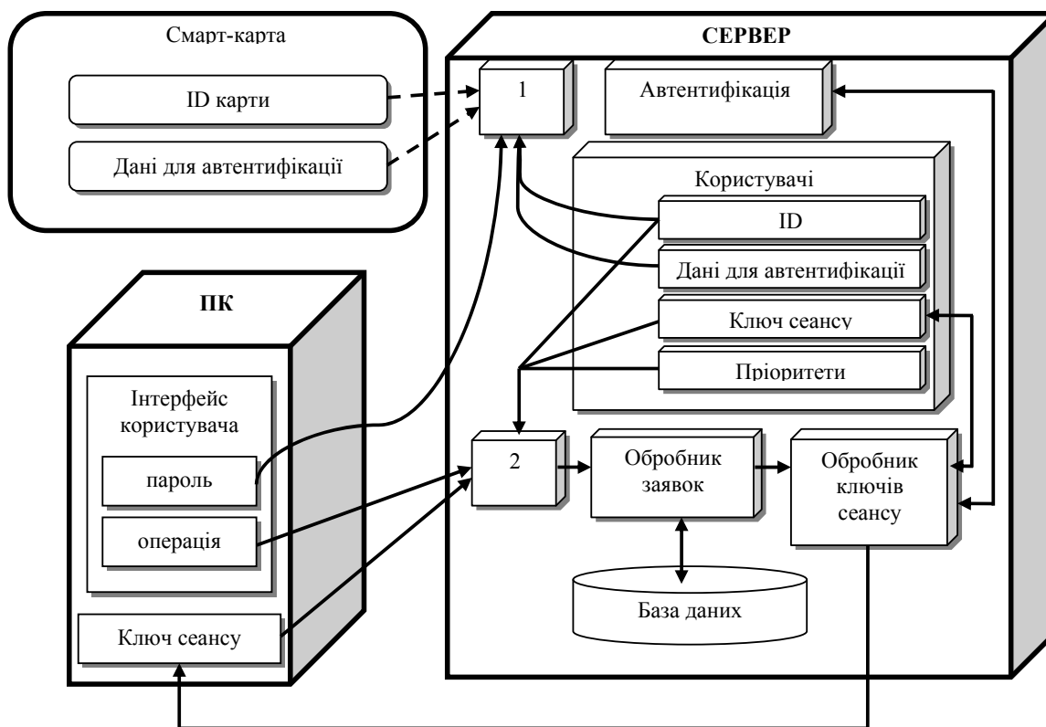
Рис. 1. Схема алгоритму доступу до інформаційної системи торгівельної мережі супермаркету на основі смарт-технологій
