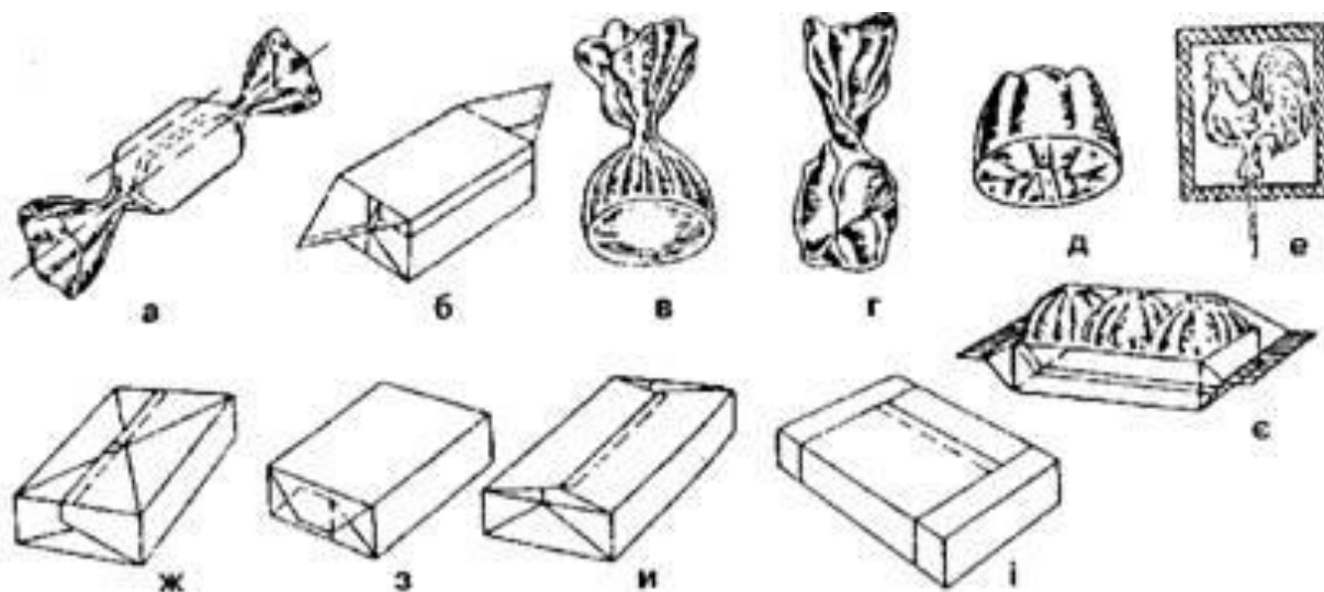
Рис. 1.3. Види загортки кондитерських виробів: а - у перегортку; б - "в носок"; в - в зтяжку; г - в "саше"; д - в обтяжку; е, е - темосклеюванням; ж - із загорткою кінців етикетки в кутик; з - з загорткою кінців етикетки із зрізаними кутками на торцях; и - в конверті; і - бандероллю
