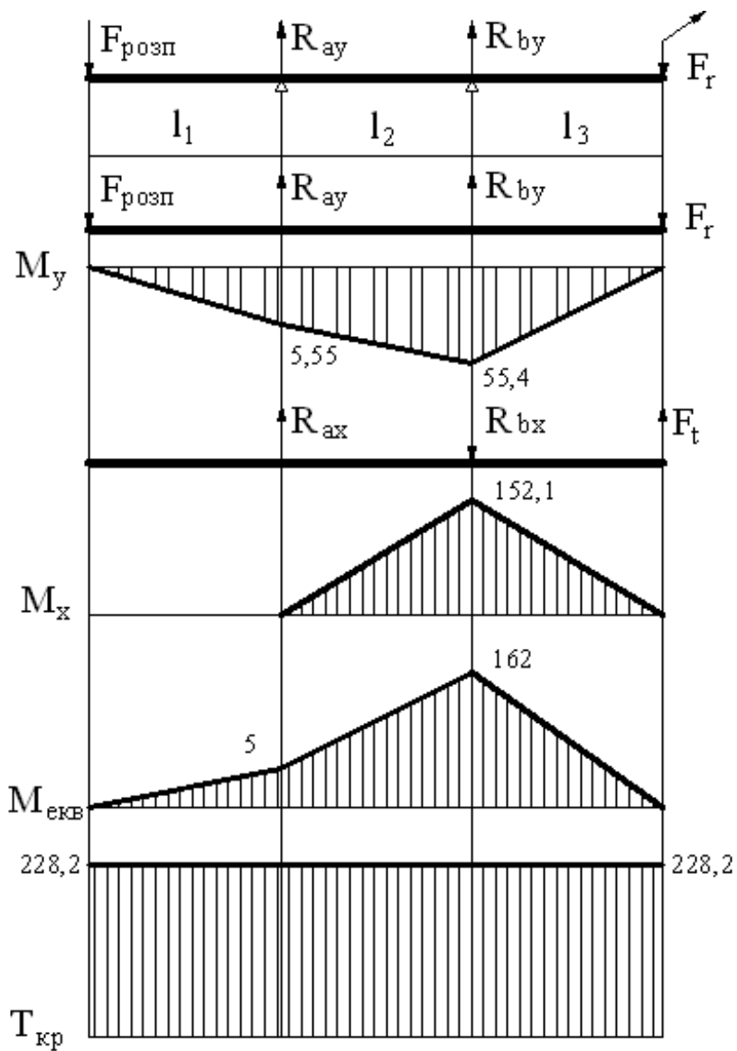
Рис. 3.2 Епюра крутних моментів
