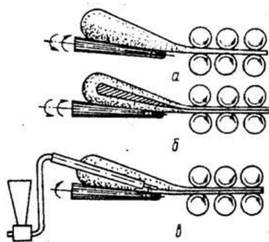
Рис. 1.1. Способи формування джгута для карамелі: а - льодяникової, б - з густою начинкою, в - з начинкою середньої густини
