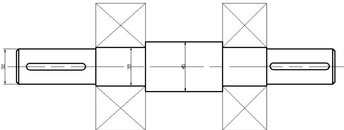
Рис.3.3 Ескіз вала
