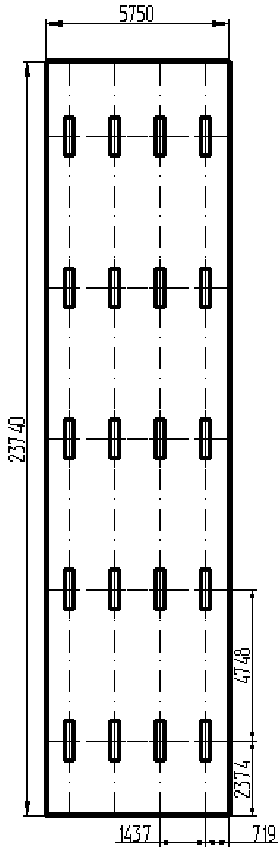
Рис.4.1 План розміщення ламп у одній половині приміщення
