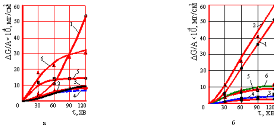
Рис. 1. Кінетика втрат маси зразків при кавітації: 1 – сталь нормалізована; 2 – Ni; 3 – \text{Ni-SiC}_{\text{нано}} ; 4 – \text{Ni-SiC}_5 ; 5 – \text{Ni-SiC}_{28} ; 6 – \text{Ni-SiC}_{50} А – жорстка вода; б – 3-відсотковий розчин NaCl
