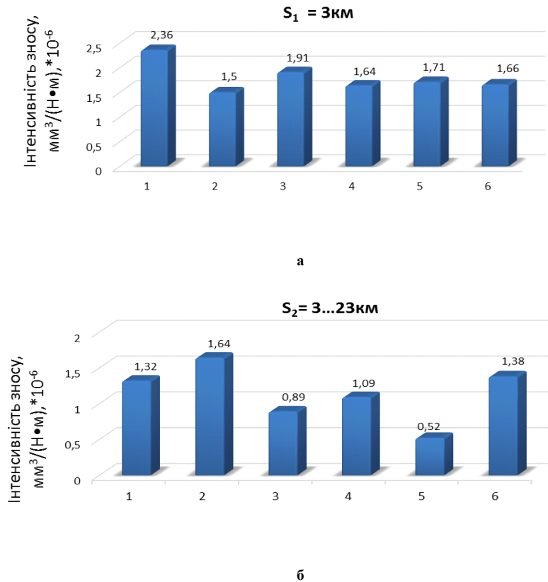
Рис. 2 – Гістограма інтенсивності зносу фторопласту, модифікованого нанопорошками діоксидів цирконію: 1 – Ф4К20; 2 – Ф4К20 + 1мас.%. (ZrO_2 + 3\%Y_2O_3, 700\text{ }^\circ\text{C}) ; 3 – Ф4К20 + 2мас.%. (ZrO_2 + 3\%Y_2O_3, 700\text{ }^\circ\text{C}) ; 4 – Ф4К20 + 1,5мас.%. (ZrO_2 + 3\%Y_2O_3, 700\text{ }^\circ\text{C}) ; 5 – Ф4К20 + 1мас.%. (ZrO_2 + 3\%Y_2O_3, \text{гідроксид}) ; 6 – Ф4К20 + 2мас.%. (ZrO_2+3\%Y_2O_3, \text{гідроксид}) ; а – перший етап досліджень; б – другий етап досліджень
