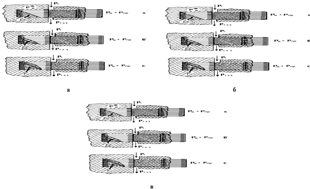
Рис. 1 – Схема розподілу тиску газу по висоті ущільнювального кільця при значенні куткового коефіцієнта: а – \beta = 1 ; б – \beta < 1 ; в – \beta > 1
