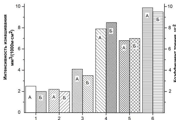
Рис.1 – Влияние материала контртела на интенсивность изнашивания (А) и коэффициент трения (Б), ( P=20 МПа, V=2,0 м/с): 1,2,3 – аморфно-кристаллическое покрытие Zr-Al-V в парах трения с образцами БрОЦС6-6-3, АО-20, 30ХГСНА; 4,5,6 – покрытие из вольфрамсодержащего сплава типа ВК-15 в парах трения с образцами БрОЦС6-6-3, АО-20, 30ХГСНА;
