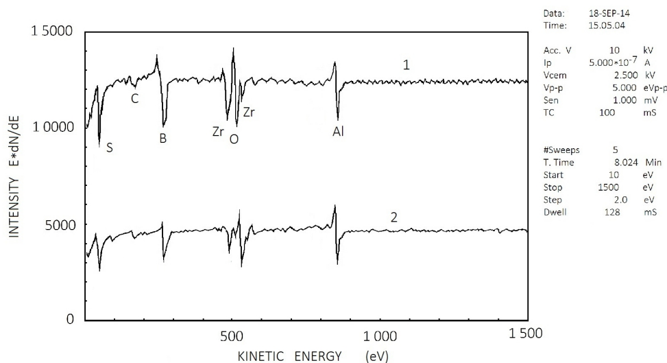
Рис. 4– Оже-спектры, снятые с поверхности (1) и после травления (2).
