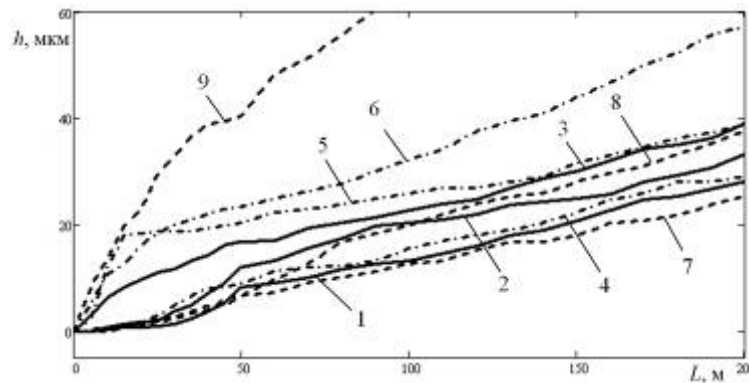
Рис. 7 – Зона припрацювання кривих зношування сталі 40Х, азотованої в тліючому розряді (цифри на кривих відповідають номерам режимів в табл.1)
