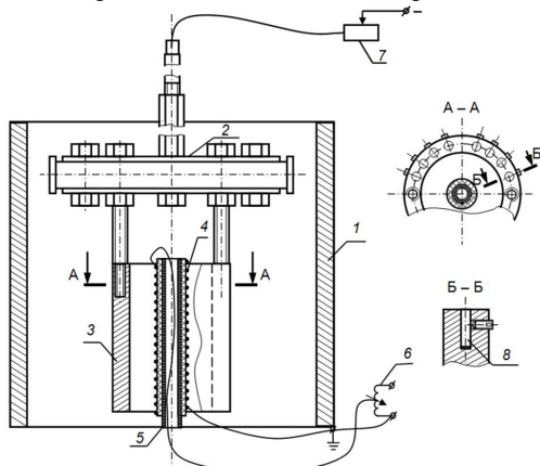
Рис. 1 – Схема пристосування для реалізації процесу азотування у тліючому розряді з автономними енергетичними параметрами:
