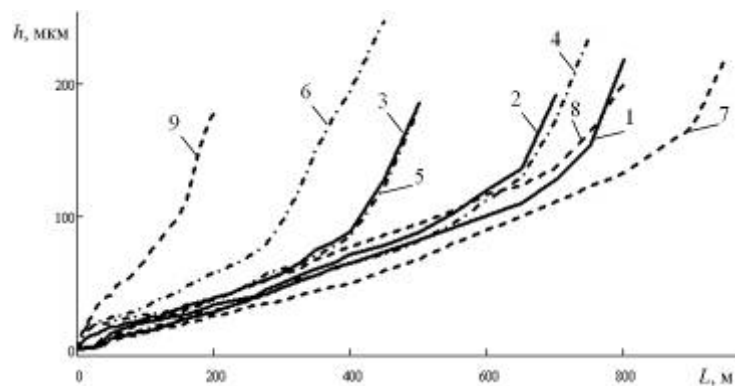
Рис. 6 – Криві зношування сталі 40Х, азотованої в тліючому розряді (цифри на кривих відповідають номерам режимів в табл. 1)
