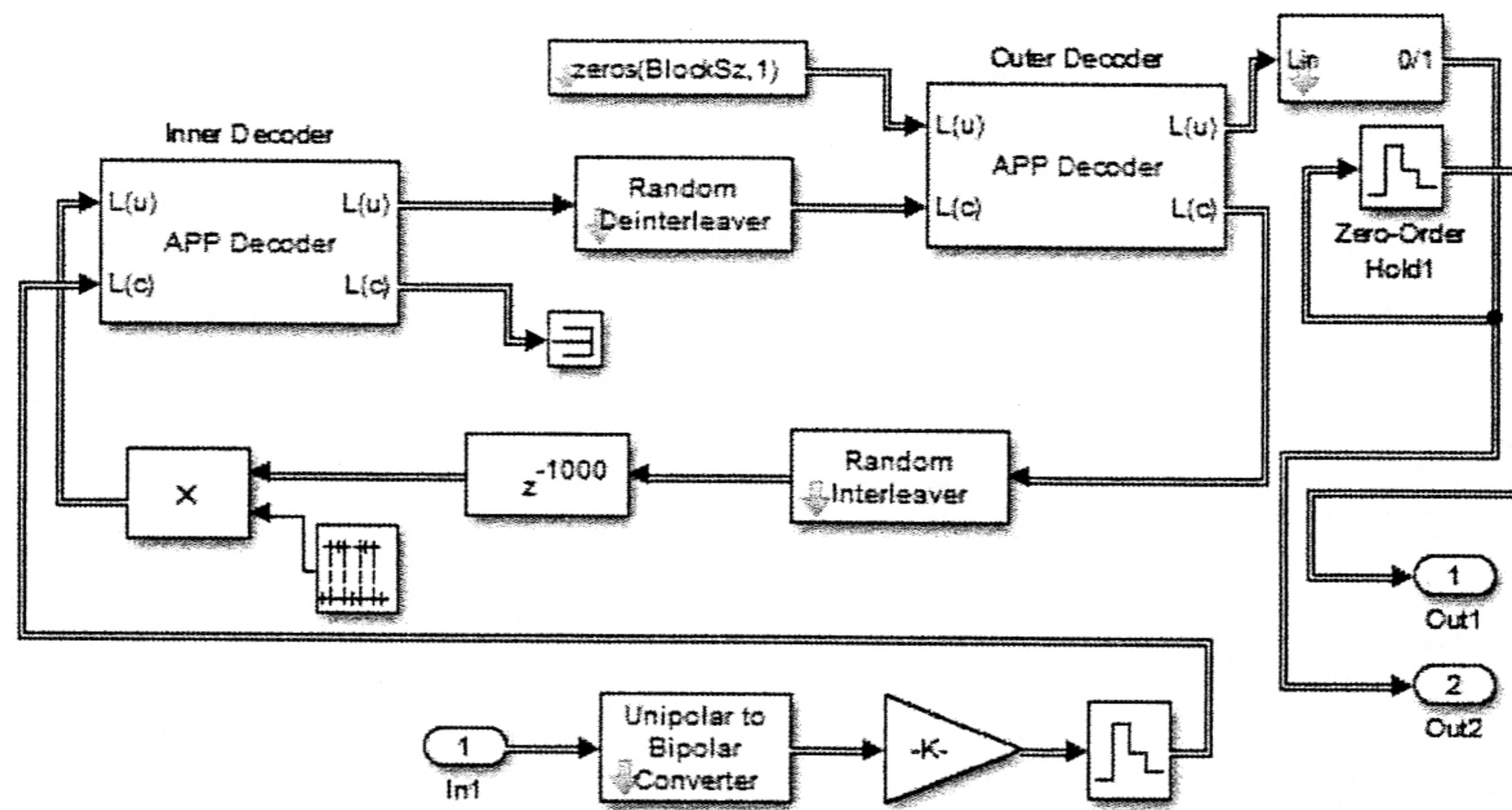
Рис. 5. Підсистема декодера турбокоду
