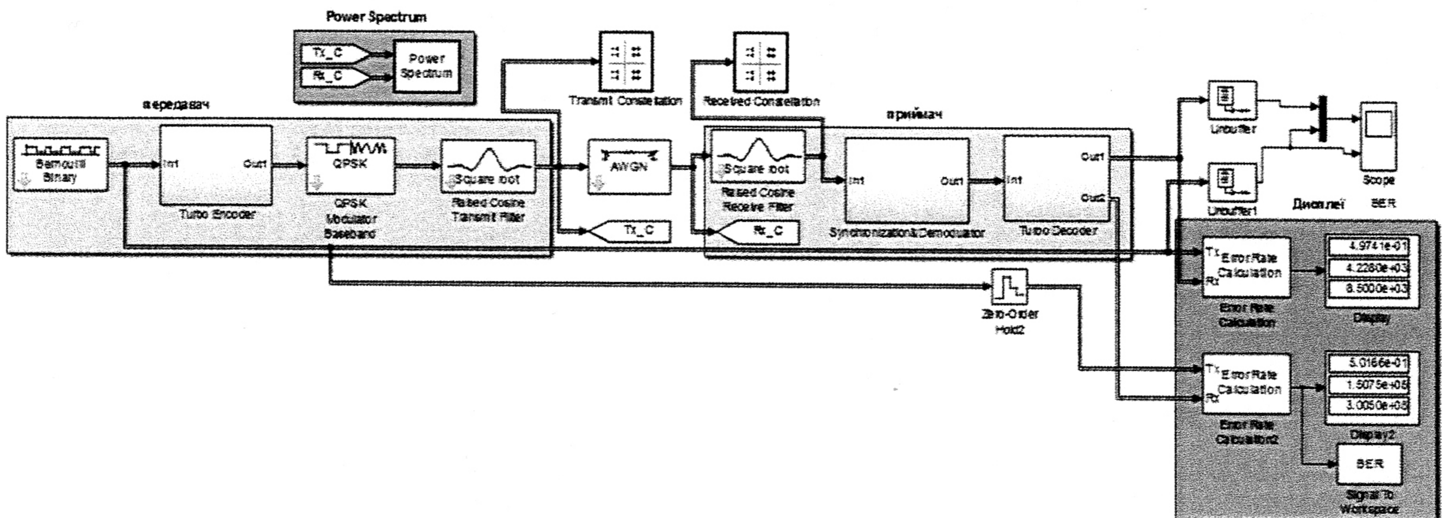
Рис. 6. Імітаційна схема для дослідження СКК на основі турбокодів і QPSK
