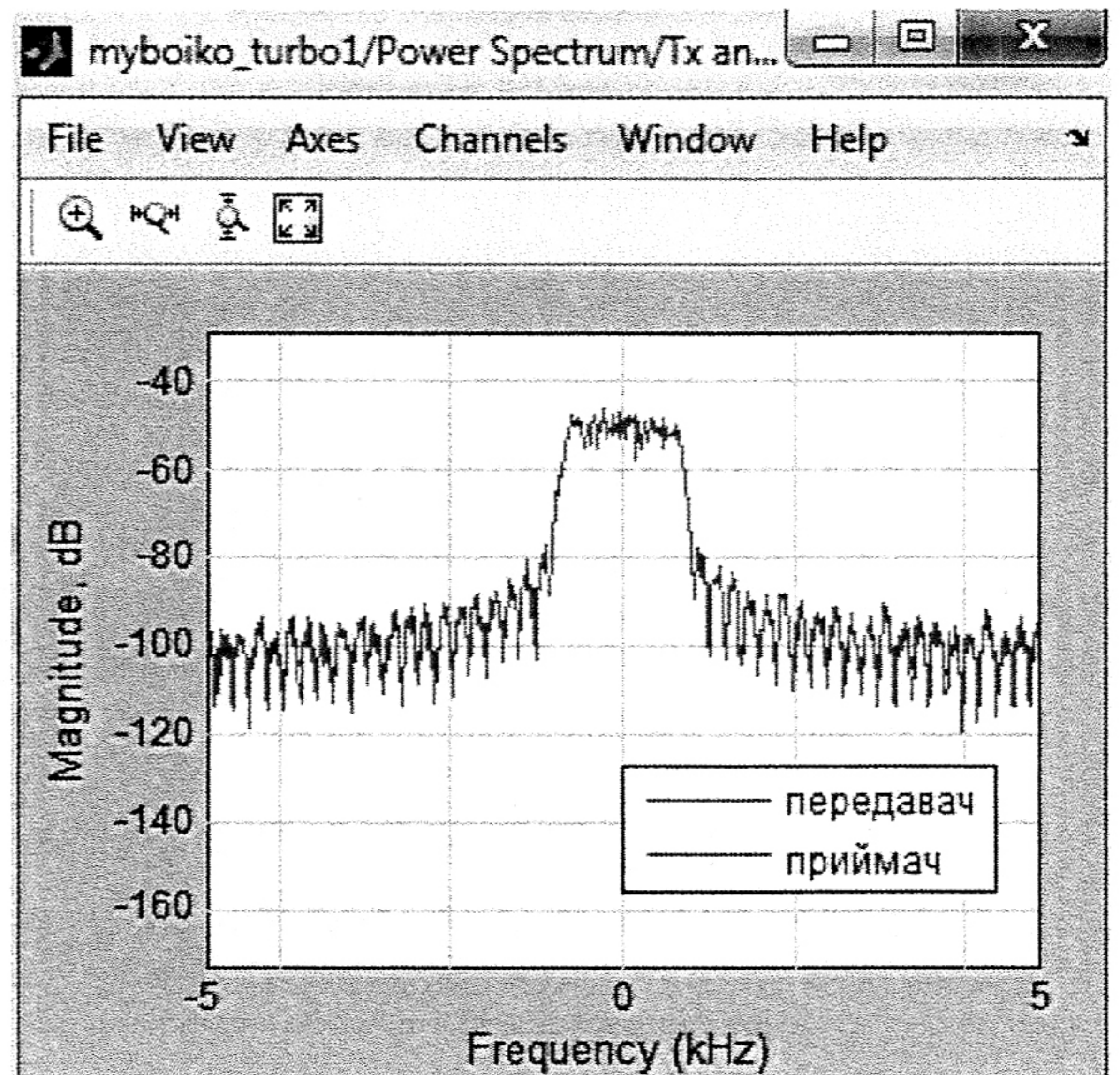
Рис. 9. Енергетичний спектр сигналу
