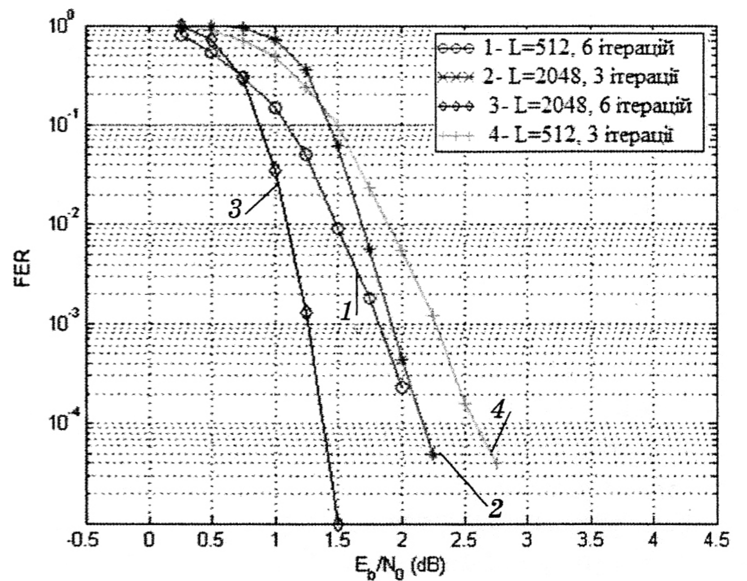
Рис. 10. Графіки залежності FER від довжини фрейма L та кількості ітерацій при турбокодуванні
