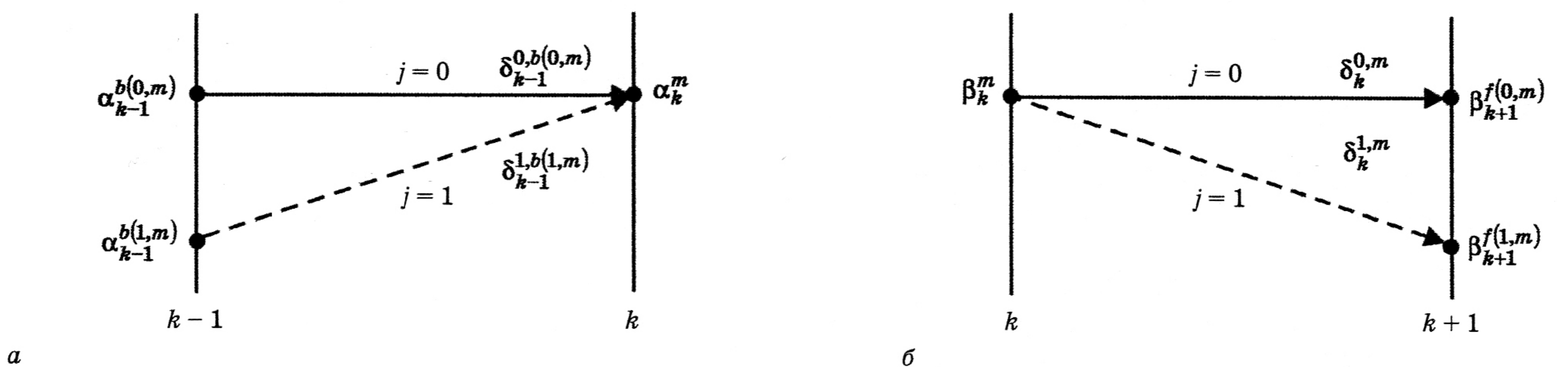
Рис. 3. Графічне подання розрахунку \alpha_k^m і \beta_k^m : а — пряма гілка стану \alpha_k^m = \alpha_{k-1}^{b(0,m)} \delta_{k-1}^{0,b(0,m)} + \alpha_{k-1}^{b(1,m)} \delta_{k-1}^{1,b(1,m)} ; б — зворотна метрика стану \beta_k^m = \beta_{k+1}^{f(0,m)} \delta_k^{0,m} + \beta_{k+1}^{f(1,m)} \delta_k^{1,m} ; \beta(j, m) — минулий стан, який відповідає вхідному j ; f(i, m) — наступний стан, який визначається вхідним j і станом m ; \delta_k^{1,m} = \pi_k^1 \exp(x_k u_k' + y_k v_k^{1,m}) — метрика гілки
