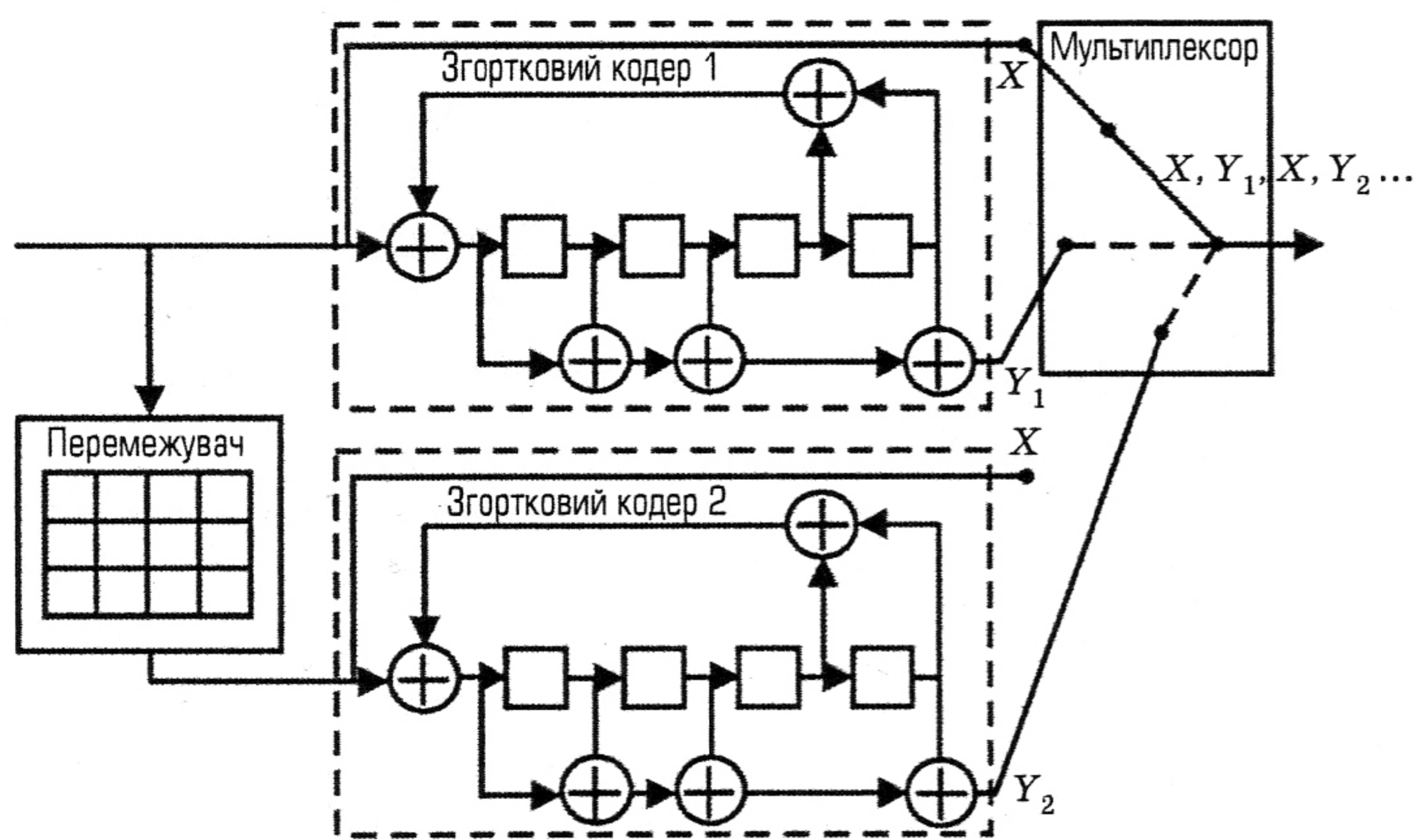
Рис. 1. Схема турбокодера
