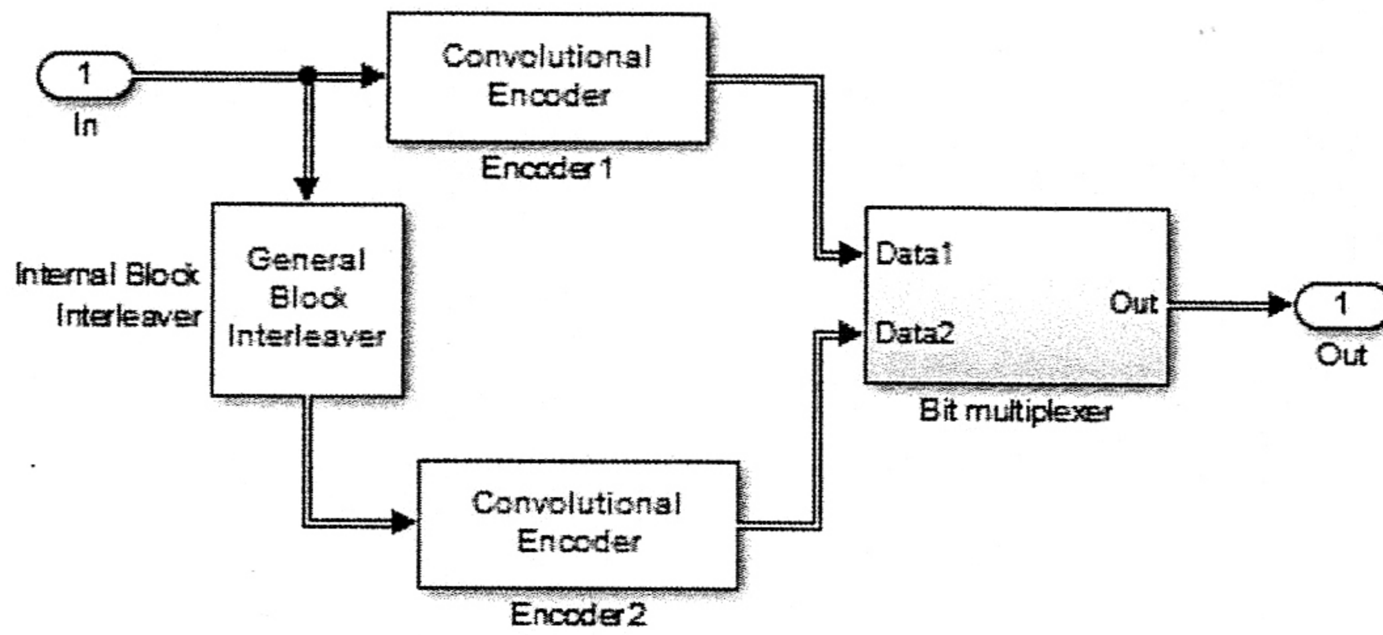
Рис. 4. Підсистема кодера турбокоду
