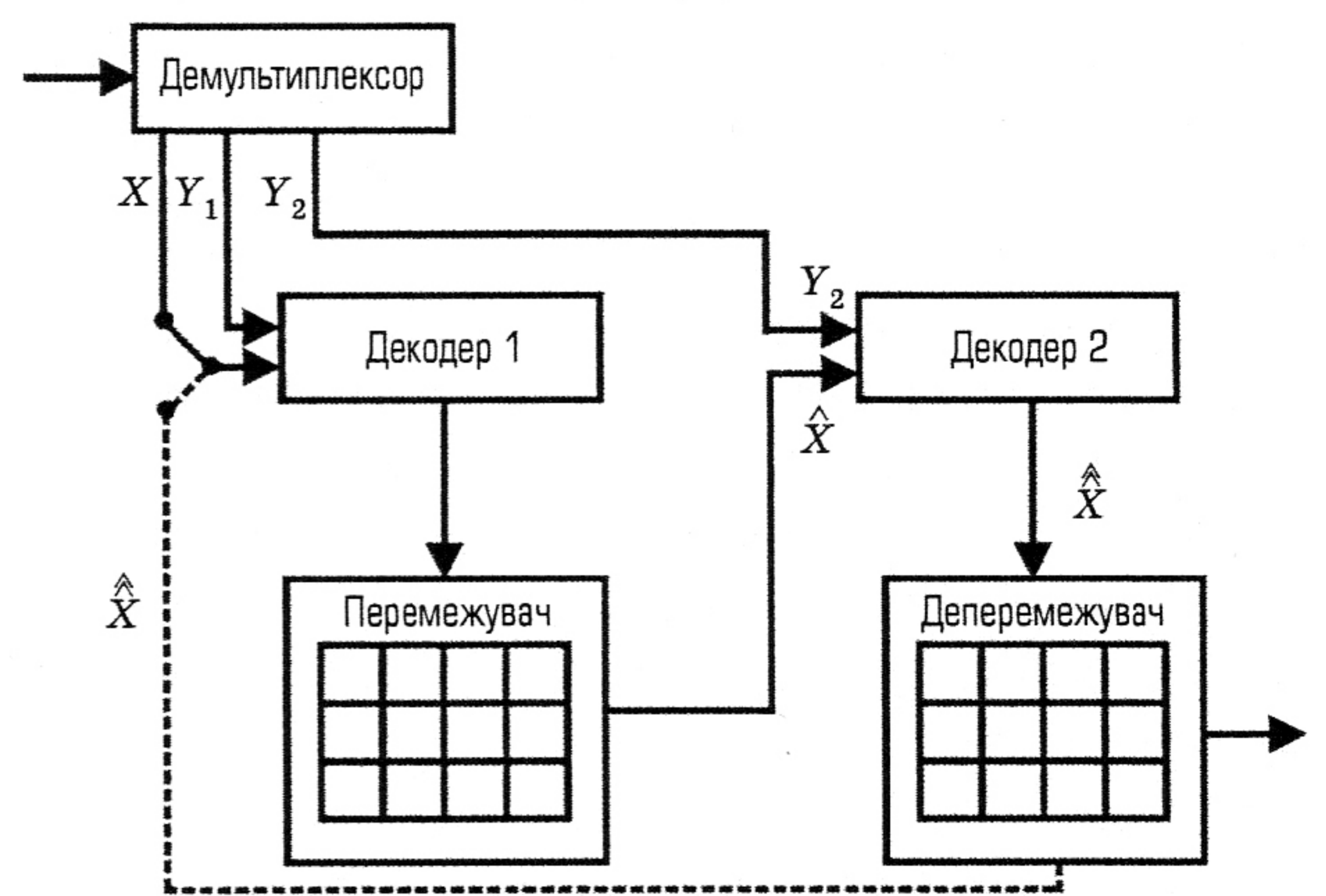
Рис. 2. Схема декодера турбокоду
