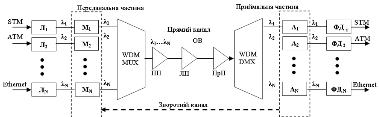
Рис. 2. Схема DWDM-системи передавання з поканалюю компенсацією поляризаційно-модової дисперсії
