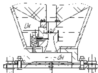
Рис. 2. Вузел вібраційного обладнання для утворення пульсуючого струменю рідини
