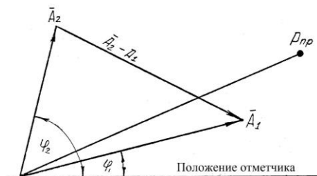
Рис. 2. Векторные построения для определения корректирующей массы
