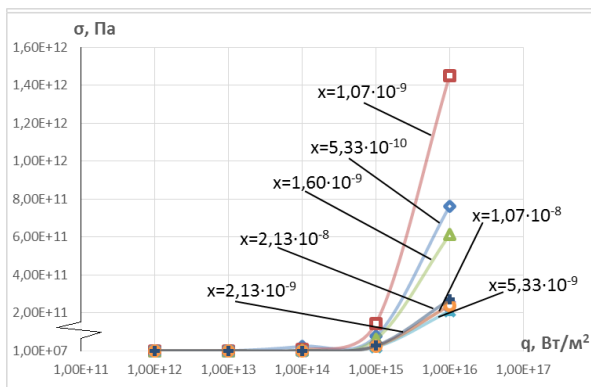
Рис. 2. Зависимость температурных напряжений в зоне действия лазерного излучения на материал “ВолКар” от плотности теплового потока на разных глубинах при времени действия t = 10^{-13} с
