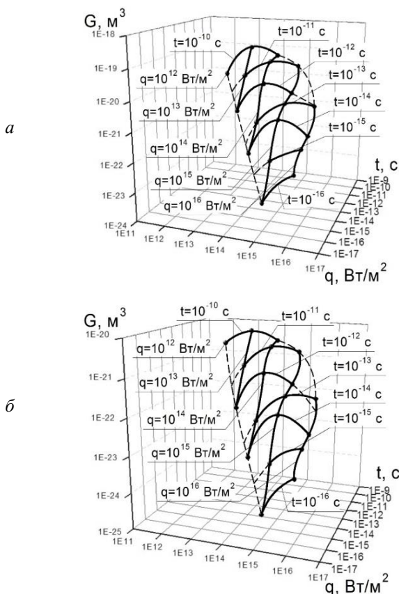
Рис. 4. Зависимость объёма нанокластера от плотности теплового потока лазерного излучения q и времени его действия t в зоне, где образуются наноструктуры (СМЧ28.48): a ) R = 10^{-6} м; б ) R = 5 \cdot 10^{-7} м
