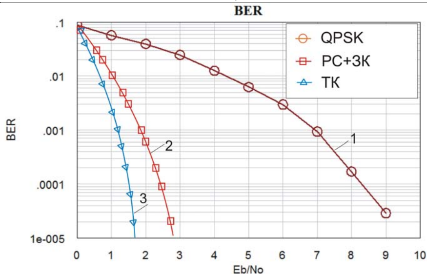
Рис. 12. Залежності бітової помилки BER від відношення сигнал/шум ( E_b / N_0 ) для AWGN каналу: 1 – для некодованої QPSK; 2 – КК (PC (255, 223), 3К (171, 133), QPSK) R=1/2 , довжина перемешувача – 5; 3 – ТК – R=1/2
