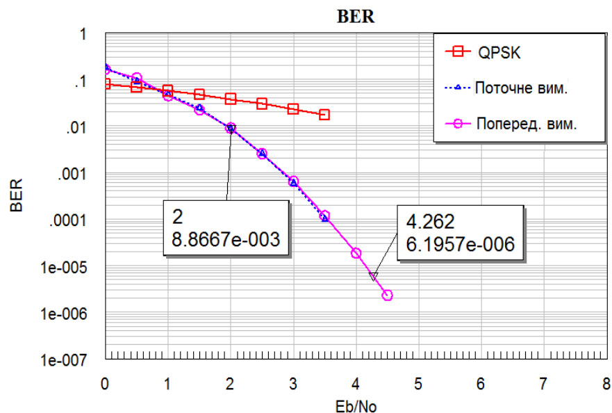
Рис. 11. Залежності біткової помилки BER від відношення сигнал/шум ( E_b / N_0 ) для AWGN каналу: ЗК (171, 133), QPSK R=1/2
