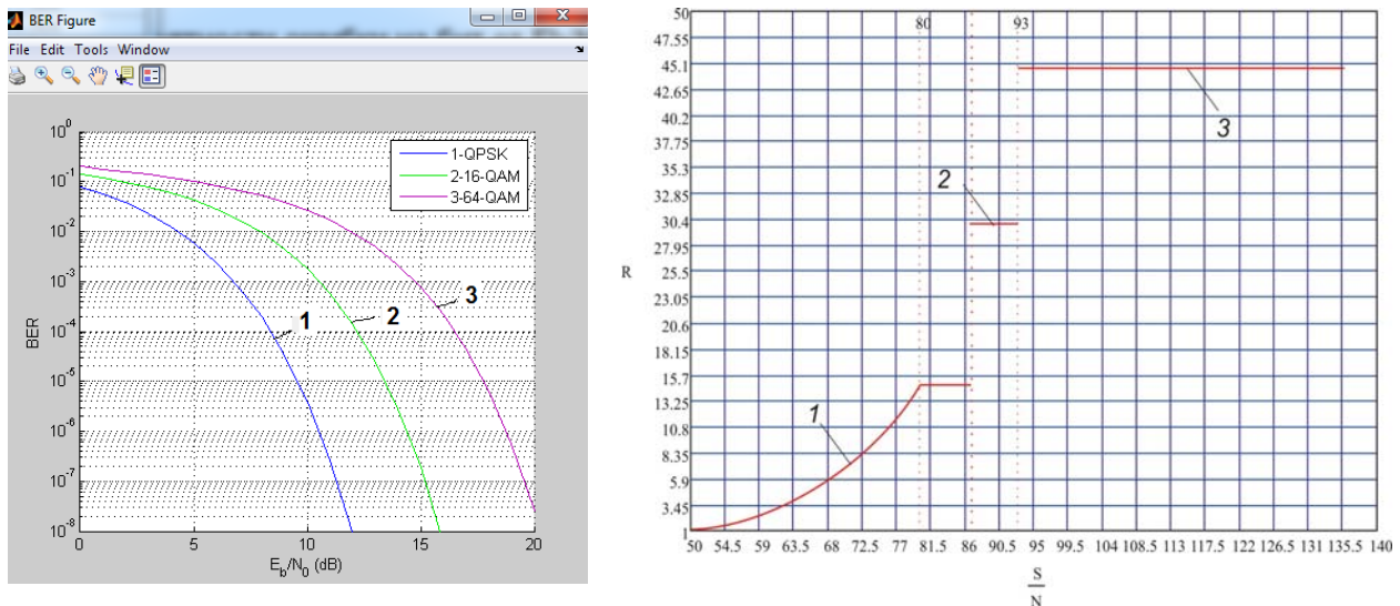
Рис. 8. Залежності ймовірності помилки на біт E_b/N_0 для модуляцій QPSK – 1, 16-QAM – 2, 3-64-QAM – 3, отримані в результаті моделювання
