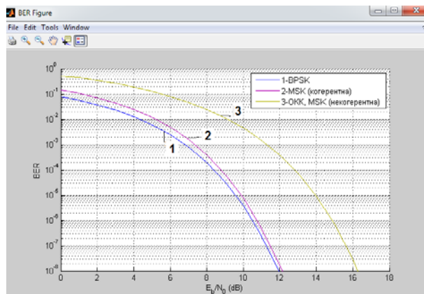
Рис. 6. Порівняння енергетичної ефективності маніпуляцій OOK, MSK, BPSK: 1- BPSK; 2 – MSK когерентна; OOK, MSK (некогерентна)
