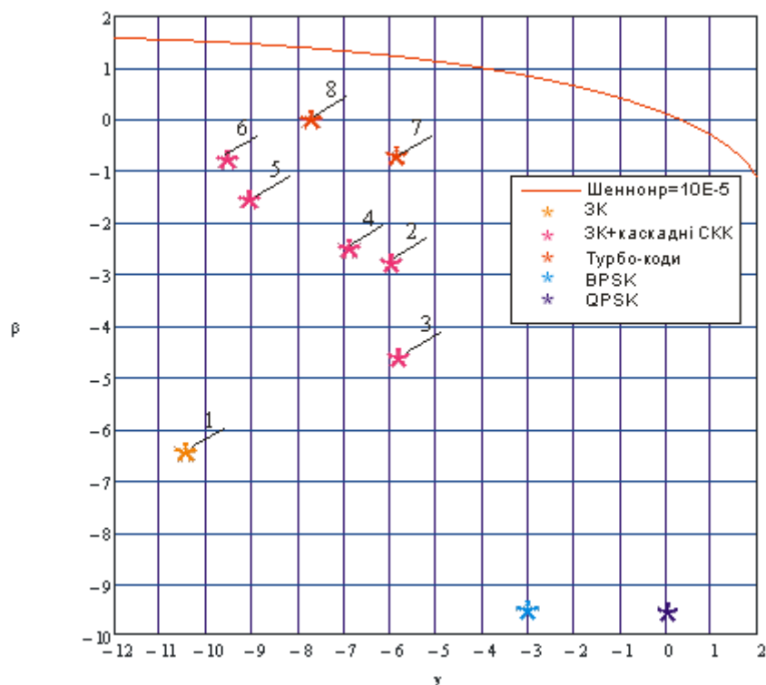
Рис. 13. Результати моделювання наближення ефективних кодів до межі Шеннона ( \beta та \gamma подано у дБ): 1 – ЗК (згортковий код); 2–6 – ЗК+каскадні СКК (згорткові коди та каскадні сигнально-кодові конструкції); 7, 8 – турбо-коди
