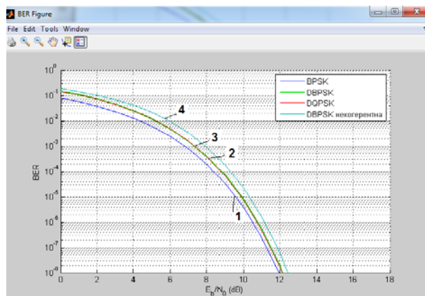
Рис. 5. Порівняння енергетичної ефективності маніпуляцій з відносним кодуванням: 1 - BPSK; 2 – DBPSK; 3 – DQPSK; 4 – DPBPSK (некогерентна)
