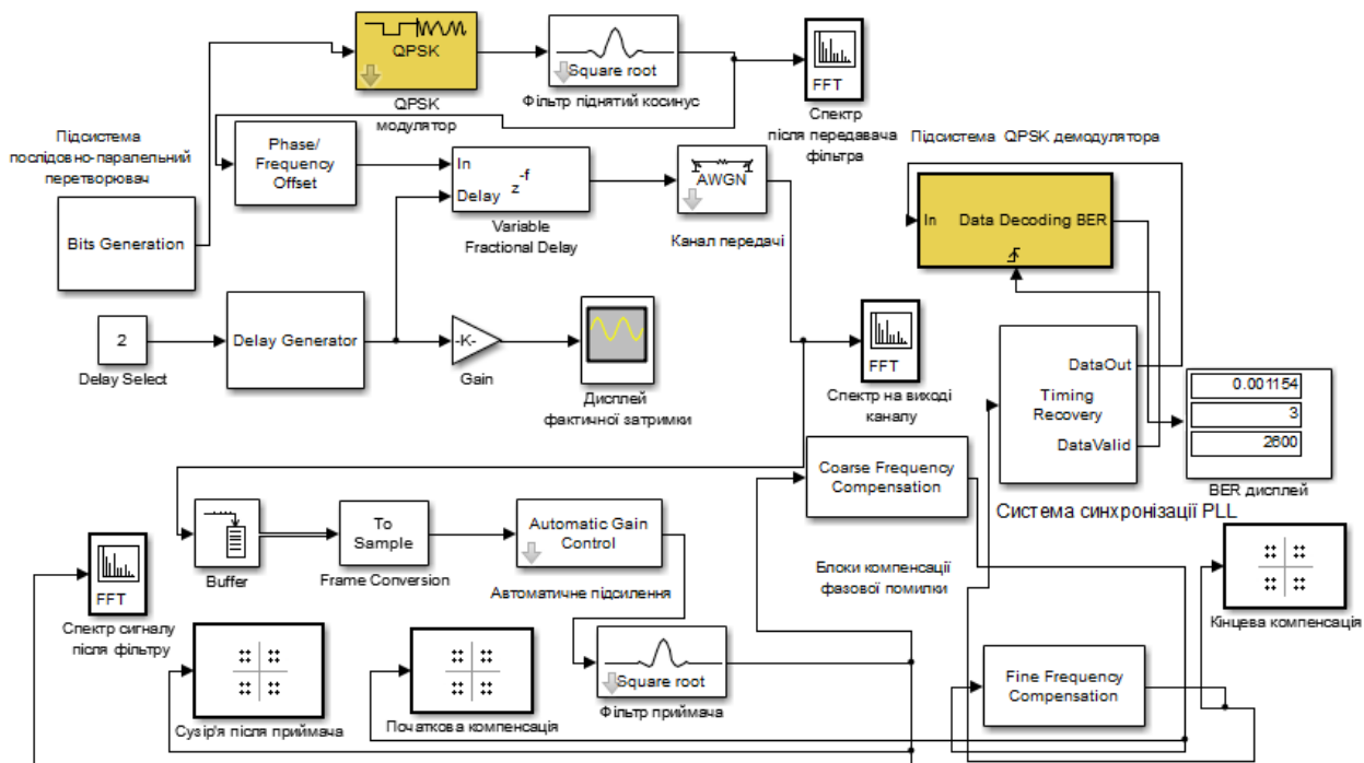
Рис. 3. Імітаційна схема передавача/приймача QPSK
