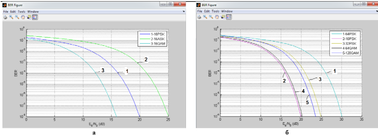
Рис. 7. Порівняння енергетичної ефективності маніпуляцій: а) 1-M-PSK; 2-M-ASK; 3-M-QAM; б) M-PSK; M-QAM
