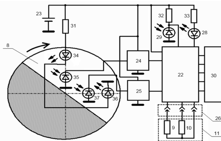
Рис. 7. Блок схема електронного відлікового пристрою роторного лічильника газу
