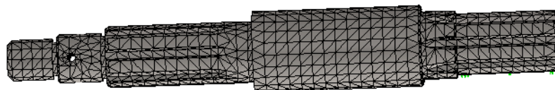
Рис. 2 – Скінченно-елементна сітка моделі валу муфти зчеплення
