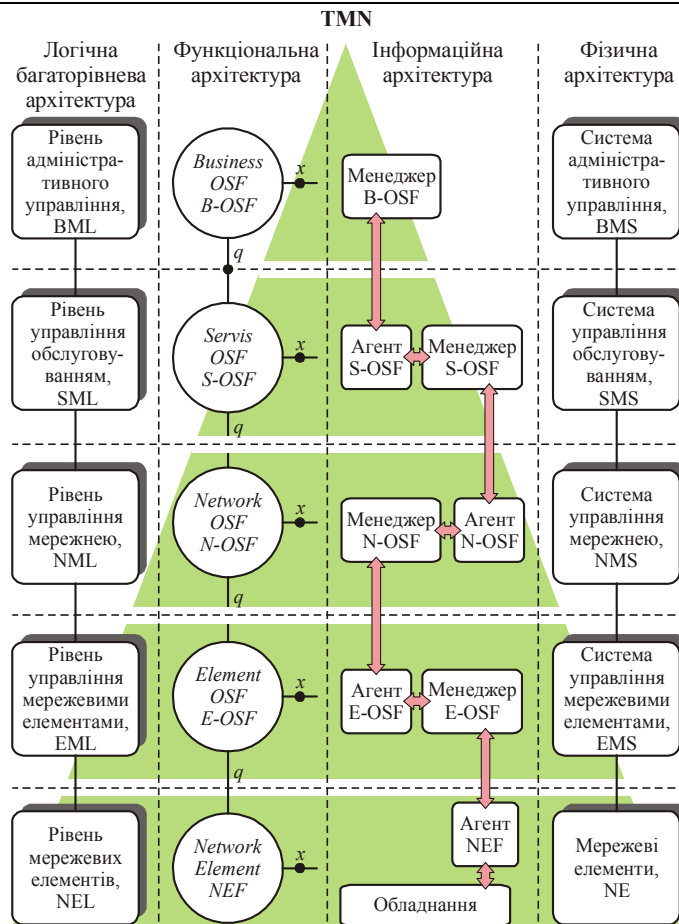
Рис. 1. Функціональна ієрархія TMN і систем підтримки
