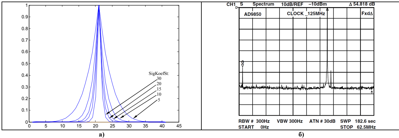
Рис. 8. Порівняння нерівномірності спектрів для (а) довільного генератора, що описується масивом SigKoef при SigKoefSt=5; 10; 15; 20; 30; (б) спектральна характеристика генератора на базі AD9850 (CLKIN = 125 MHz/fOUT = 41 MHz) [8]
