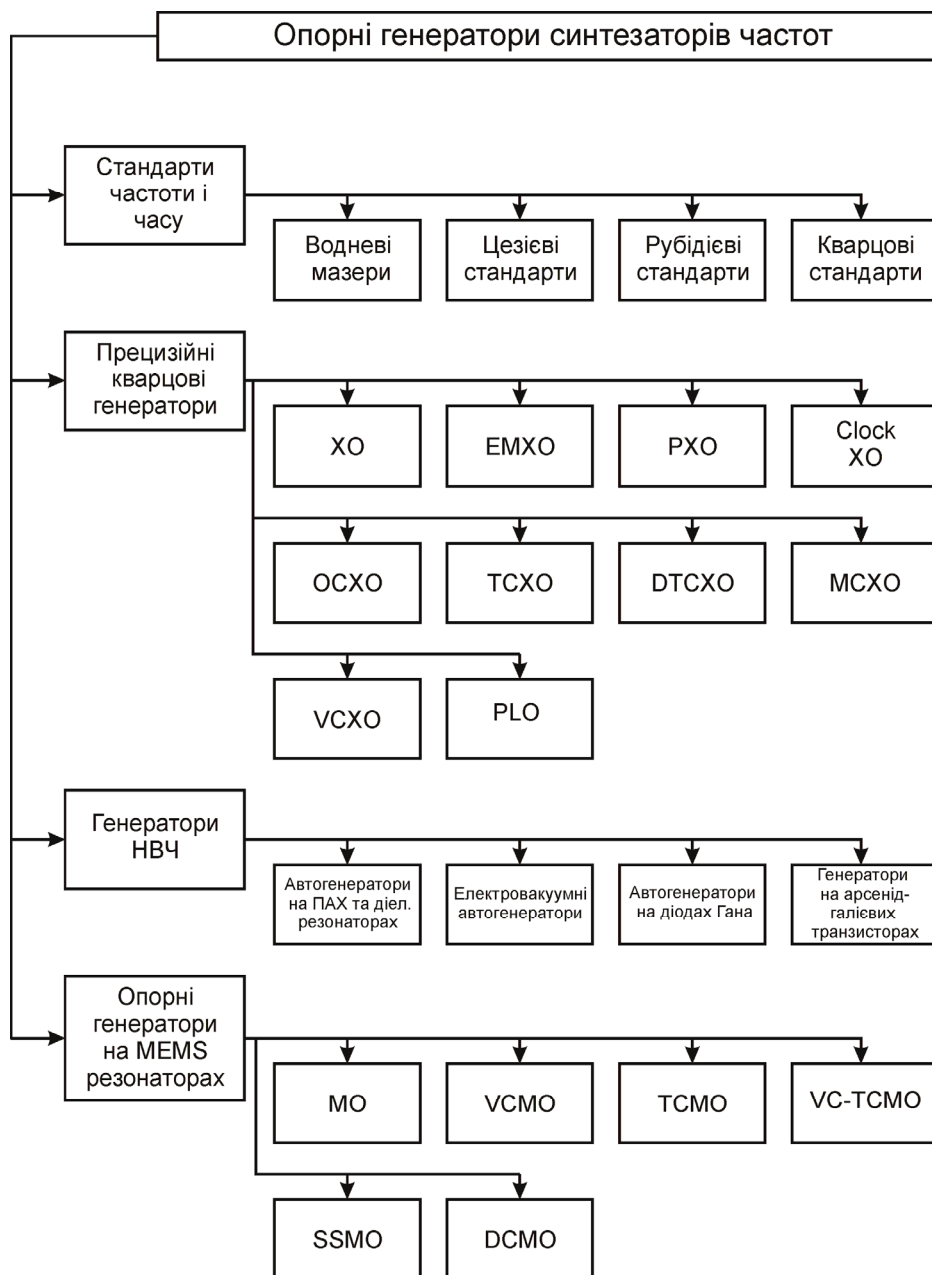
Рис. 1. Класифікація опорних автогенераторів систем синтезу частот: звичайні кварцові генератори (Crystal oscillator - XO); вакуумовані мініатюрні (Evacuated miniature - EMХО); прецизійні (Precision... -РХО); тактові (Clock XO); термостабілізовані (Oven controlled... - ОСХО); термокомпенсовані (Temperature compensated... - ТСХО); з цифровою компенсацією (Digitally compensated... - DТСХО); з мікропроцесорною компенсацією (Microprocessor compensated... - МСХО);керовані напругою за частотою (Voltage controlled...- VCХО); синхронізовані за фазою (Phase locked...- PLO)
