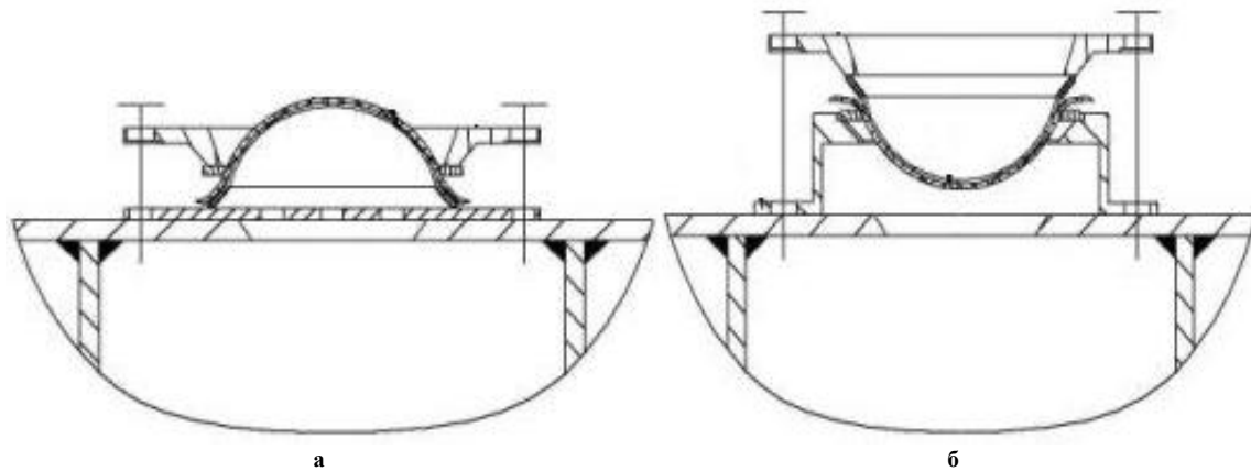
Рис. 1. Схема кріплення формуального елемента а – опуклий формувальний елемент; б – ввігнутий формувальний елемент
