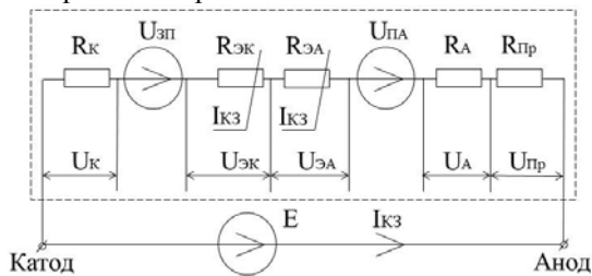
Рис. 1. Нелинейная эквивалентная схема замещения, моделирующая параметры в процессе непрерывного контроля защитного потенциала ЭНВ
