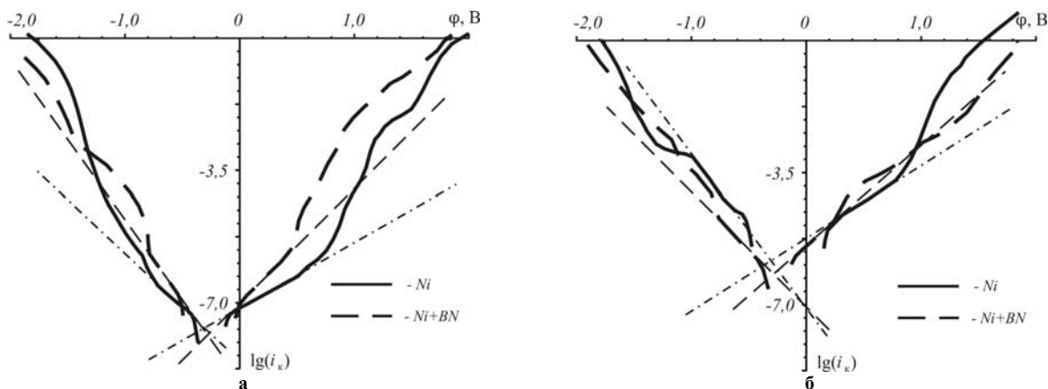
Рис. 2. Залежність функції логарифму густини струму від потенціалу а - зразки без відпалу; б - зразки відпалені при температурі 760^\circ\text{C} протягом однієї години
