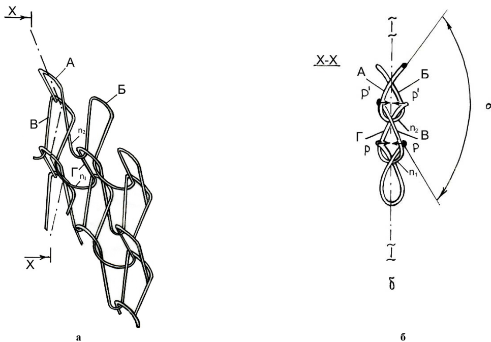
Рис. 4. Графічна схема структури повного двовиворітного ластика
