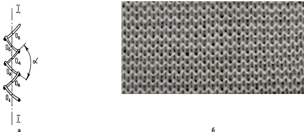
Рис. 1. Графічна схема структури (а) та зразок (б) двовиворітної гладі
