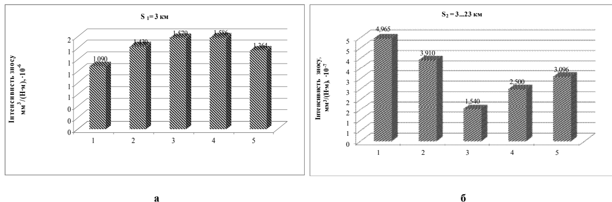
Рис. 2 – Гістограма інтенсивності зносу матеріалу Ф4К10ВВ10, модифікованого нанопорошком оксиду цирконію ZrO_2 + 3\% Y_2O_3, 700^\circ C .
