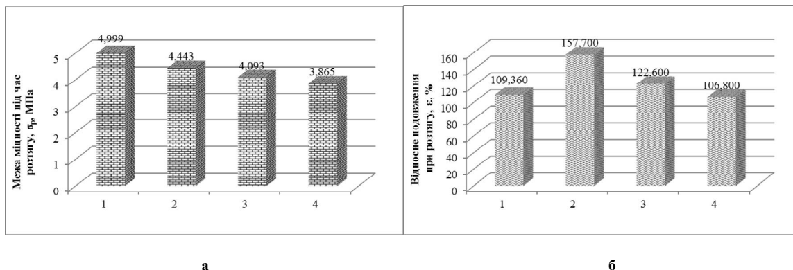
Рис. 3 – Гістограма межі міцності під час розтягу (а) і відносного подовження при розтягу (б) антифрикційних матеріалів: 1 – Ф4К10ВВ10; 2 – Ф4К10ВВ10 + 1мас.%(ZrO 2 + 3 % Y 2 O 3 , 700 °С); 3 – Ф4К10ВВ10 + 2мас.%(ZrO 2 + 3 % Y 2 O 3 , 700°С); 4 – Ф4К10ВВ10 + 3мас.%(ZrO 2 + 3 % Y 2 O 3 , 700°С)
