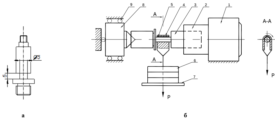
Рис. 1 – Образец (а) и схема машины трения (б): 1 – электродвигатель; 2 – зажимное устройство (цанга); 3 – образец; 5 – абразивная прокладка; 6 – гири; 7 – основание подвеса; 4 – контргтело; 8 – подвижная осевая опора (центрирующая); 9 – шарикоподшипниковые опоры
