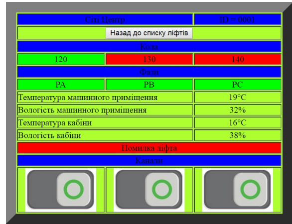
Рис. 6. Вкопіровка вікна дистанційного моніторингу стану ліфта
