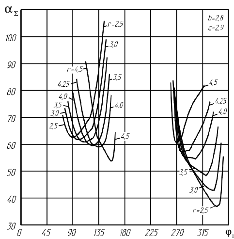
Рис. 6. Діаграма зміни тривалості зупинки вихідної ланки механізму
