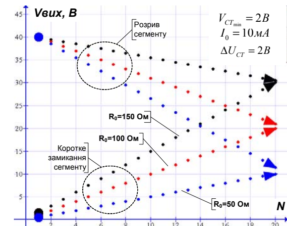
Рис. 3. Сукупна діаграма залежності вхідної напруги методу нелінійної реакції для випадку холостого ходу та замикання сегменту
