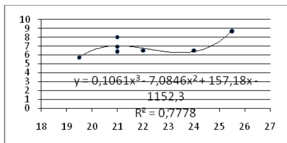
Рис. 1. Графік залежності радіуса кривизни плеча від кута нахилу плечового схилу для фігур з O_{г3} = 80 см
