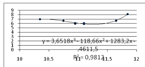
Рис. 2. Графік залежності радіуса кривизни плеча від ширини плечового схилу для фігур з O_{г3} = 84 см
