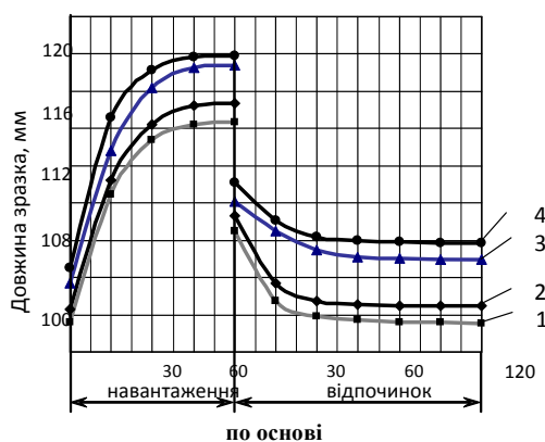
Рис. 3. Релаксаційні процеси досліджуваного матеріалу в адсорбційно-активних середовищах (середовище 1–4 відповідно таблиці 1)
