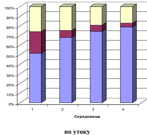
Рис. 2. Складові повної деформації досліджуваного матеріалу в рідинно-активних середовищах (середовище 1–4 відповідно таблиці 1)
