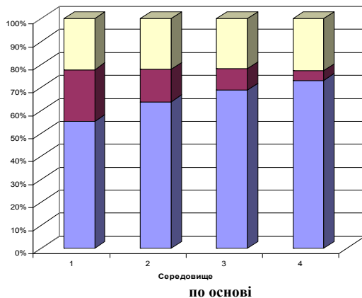
Рис. 2. Складові повної деформації досліджуваного матеріалу в рідинно-активних середовищах (середовище 1–4 відповідно таблиці 1)
