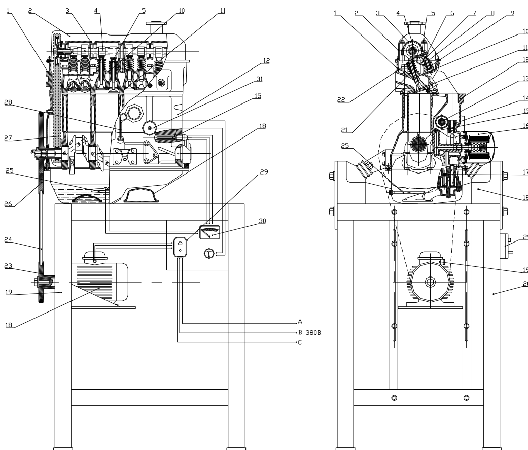
Рис. 2. Схема стенда
