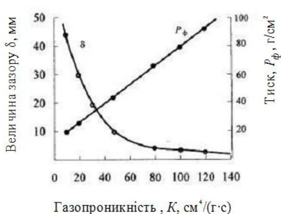
Рис. 3. Залежність тиску P_\phi і величини зазору \delta від газопроникності форми
