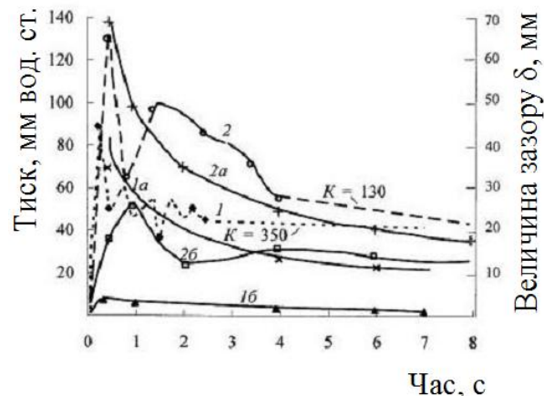
Рис. 4. Кінетика тиску і величини зазору \delta 1,2 – експериментальні тиски P_\phi , 1a, 2a – розрахункові P_\phi ; 1б,2б – розрахункова величина зазору \delta
