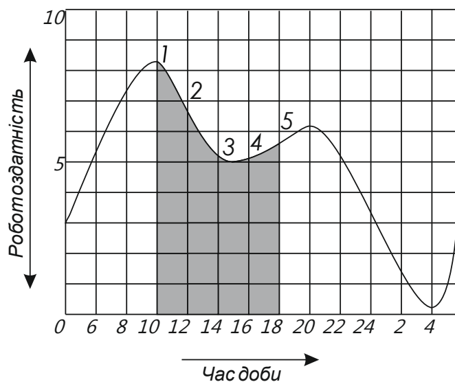
Рис. 1. Графік СКП-функції
