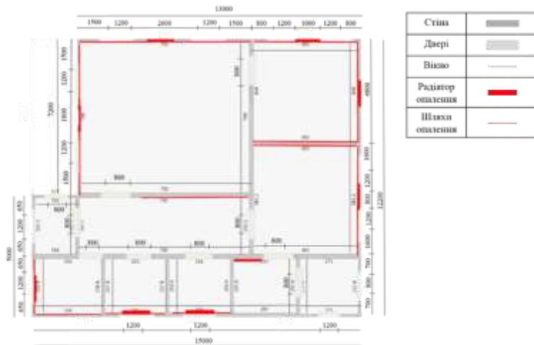
Рисунок 3.5 – План опалення
