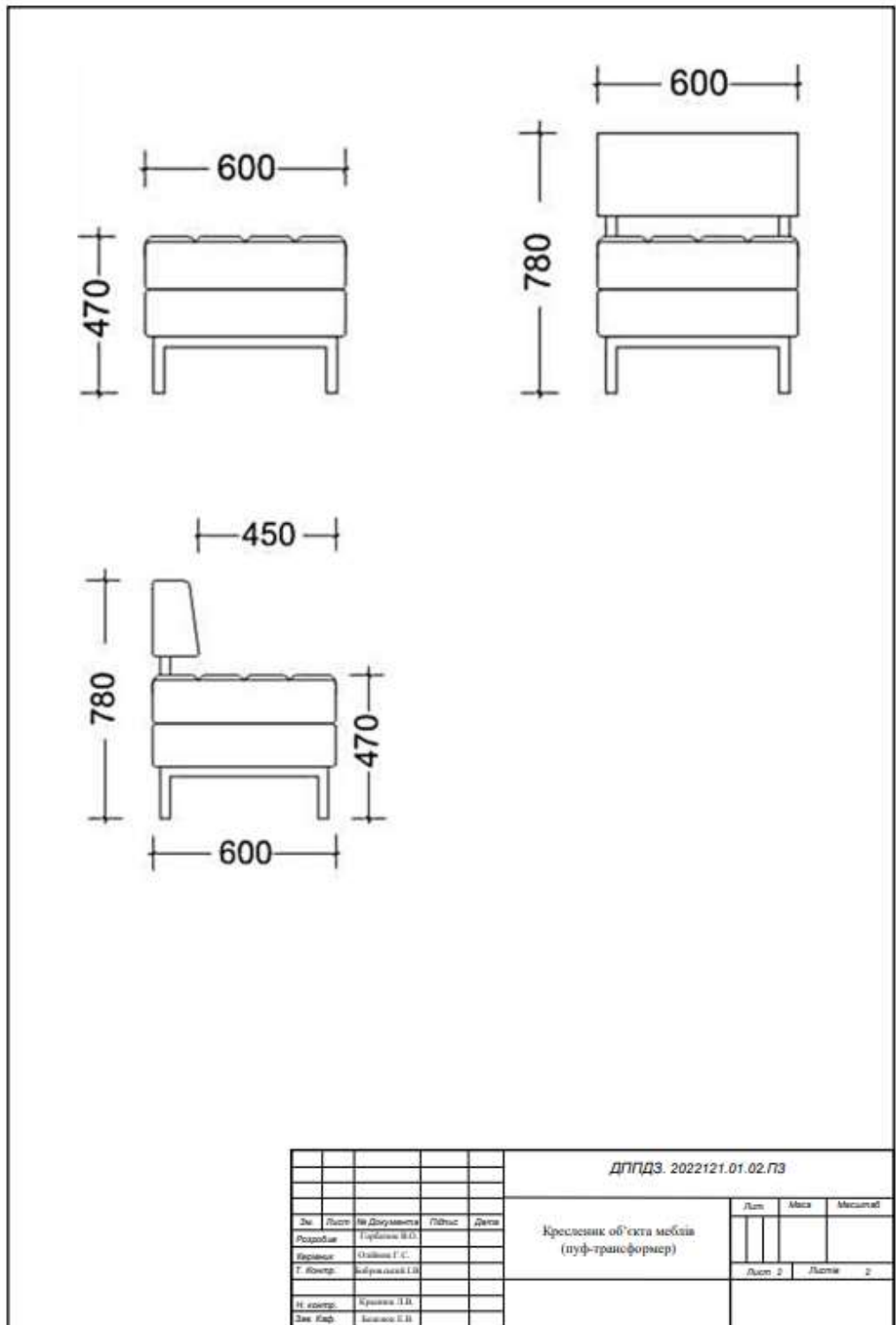
Рисунок А10 – Креслення об'єкта меблів (пуф-трансформер)
