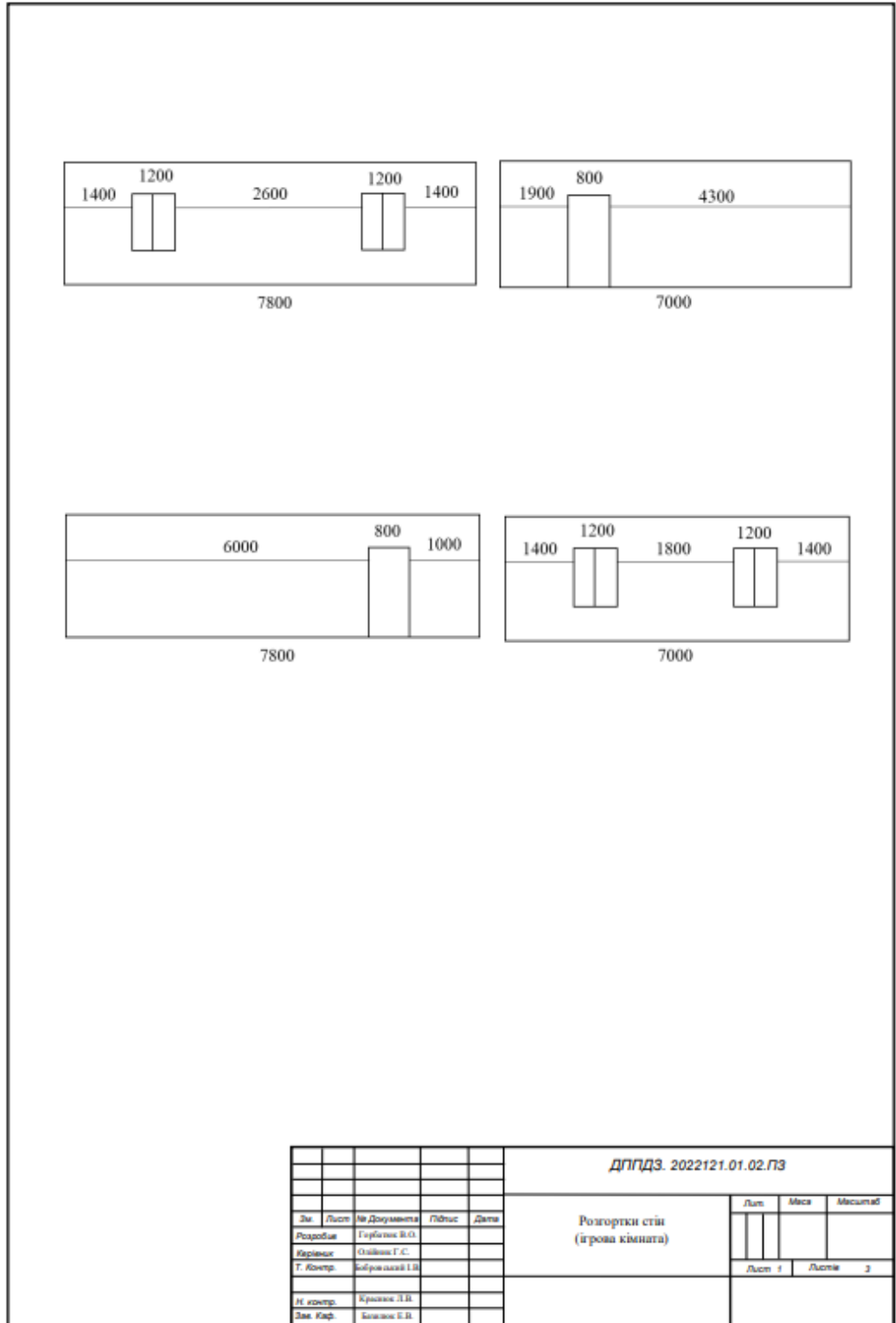
Рисунок А6 – Розгортки стін (ігрова кімната)
