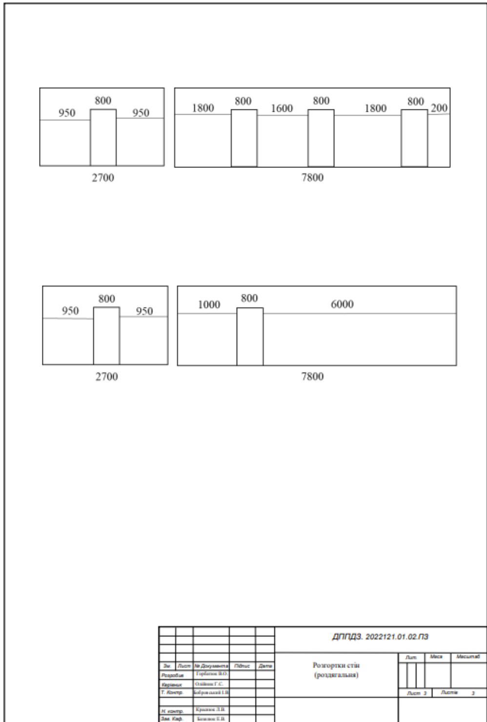
Рисунок А8 – Розгортки стін (роздягальня)
