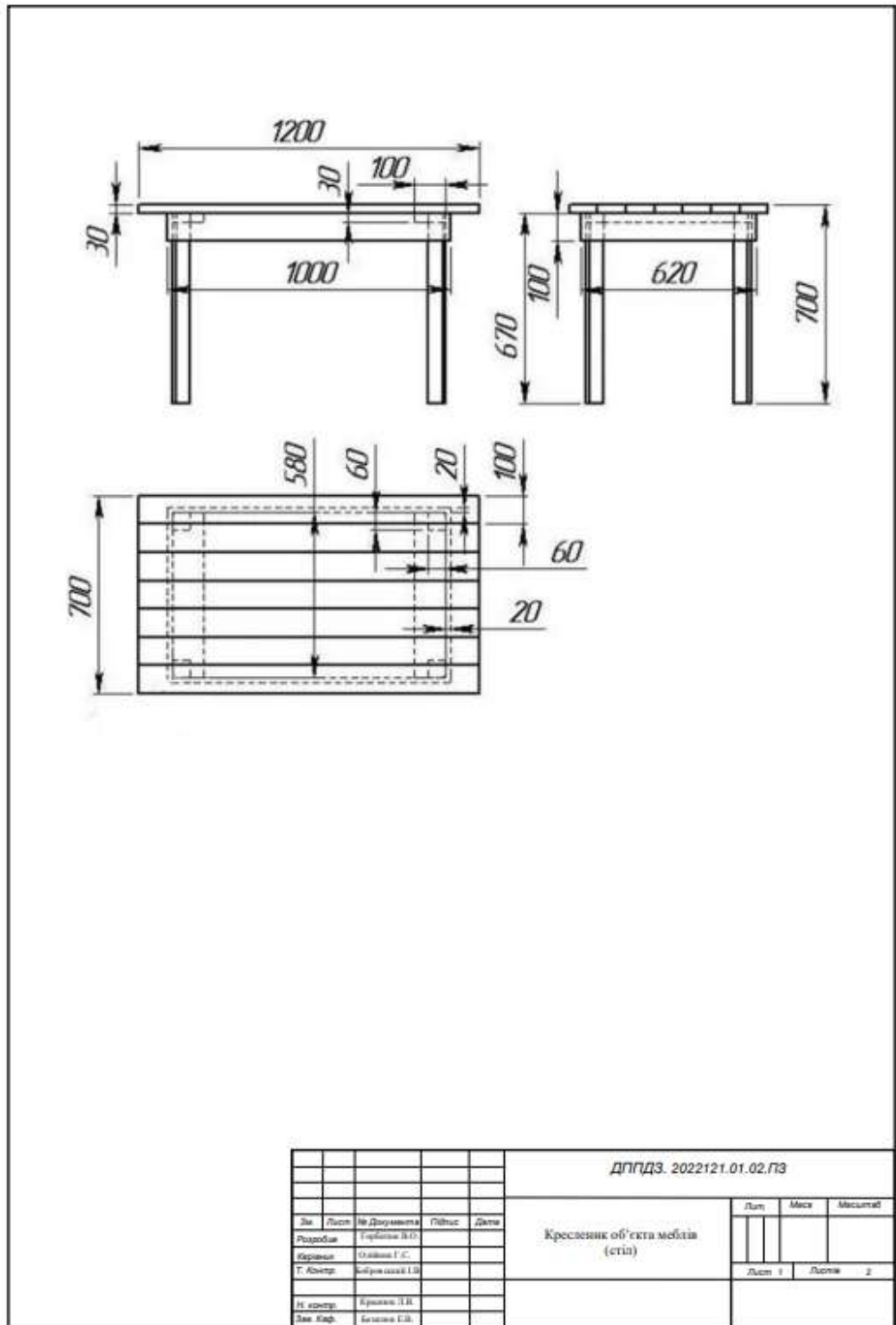
Рисунок А9 – Кресленик об'єкта меблів (стіл)
