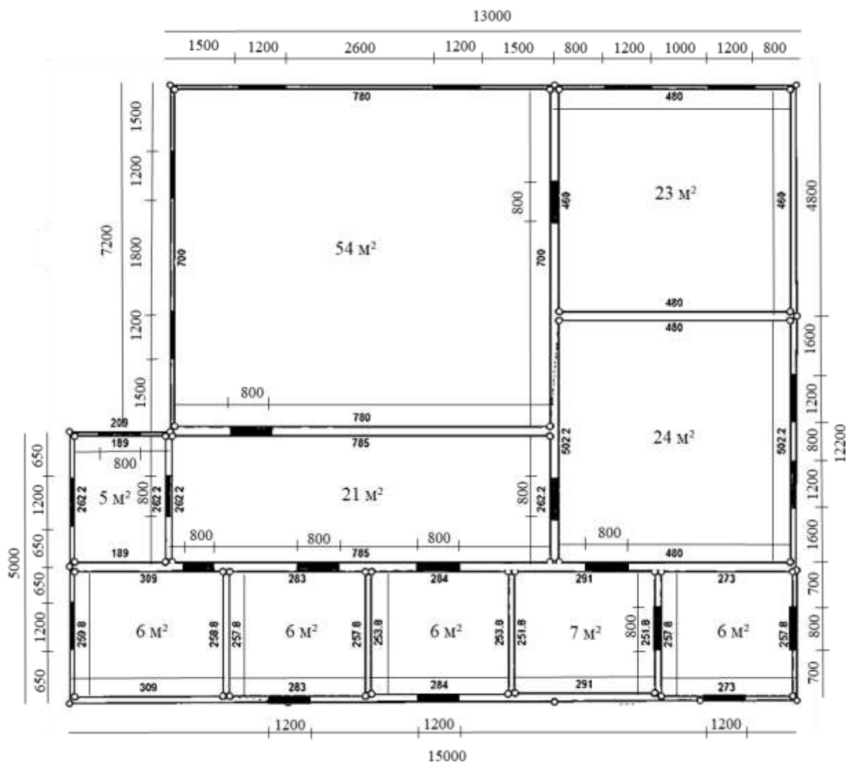
Рисунок 3.1 – Обмірний план приміщення
