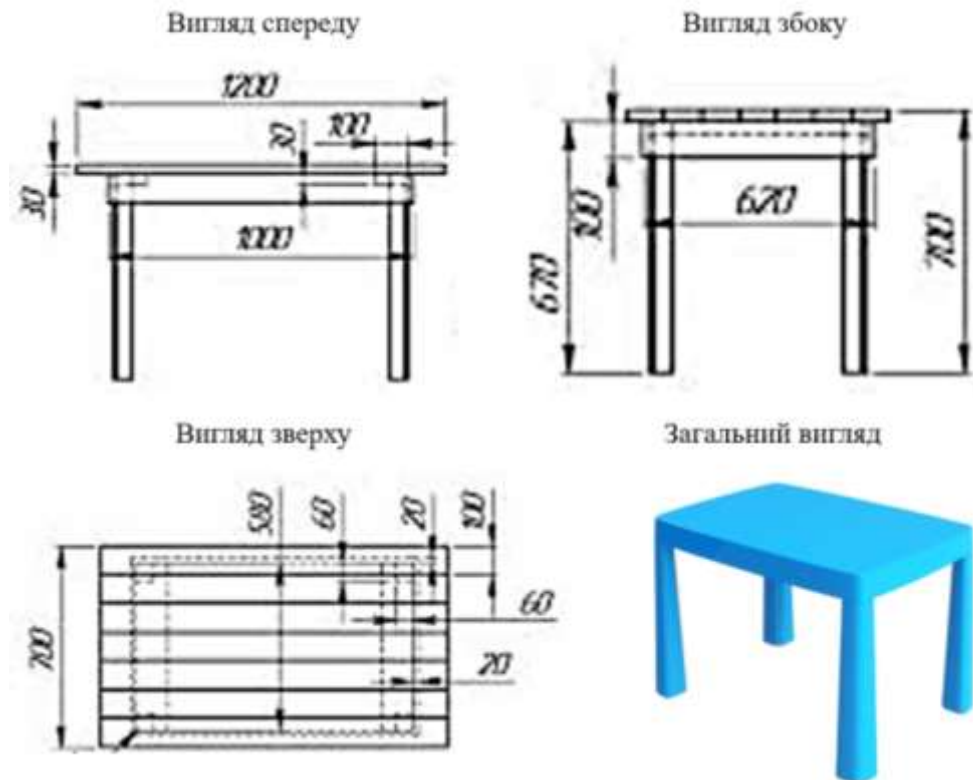
Рисунок 3.11 – Кресленик стола
