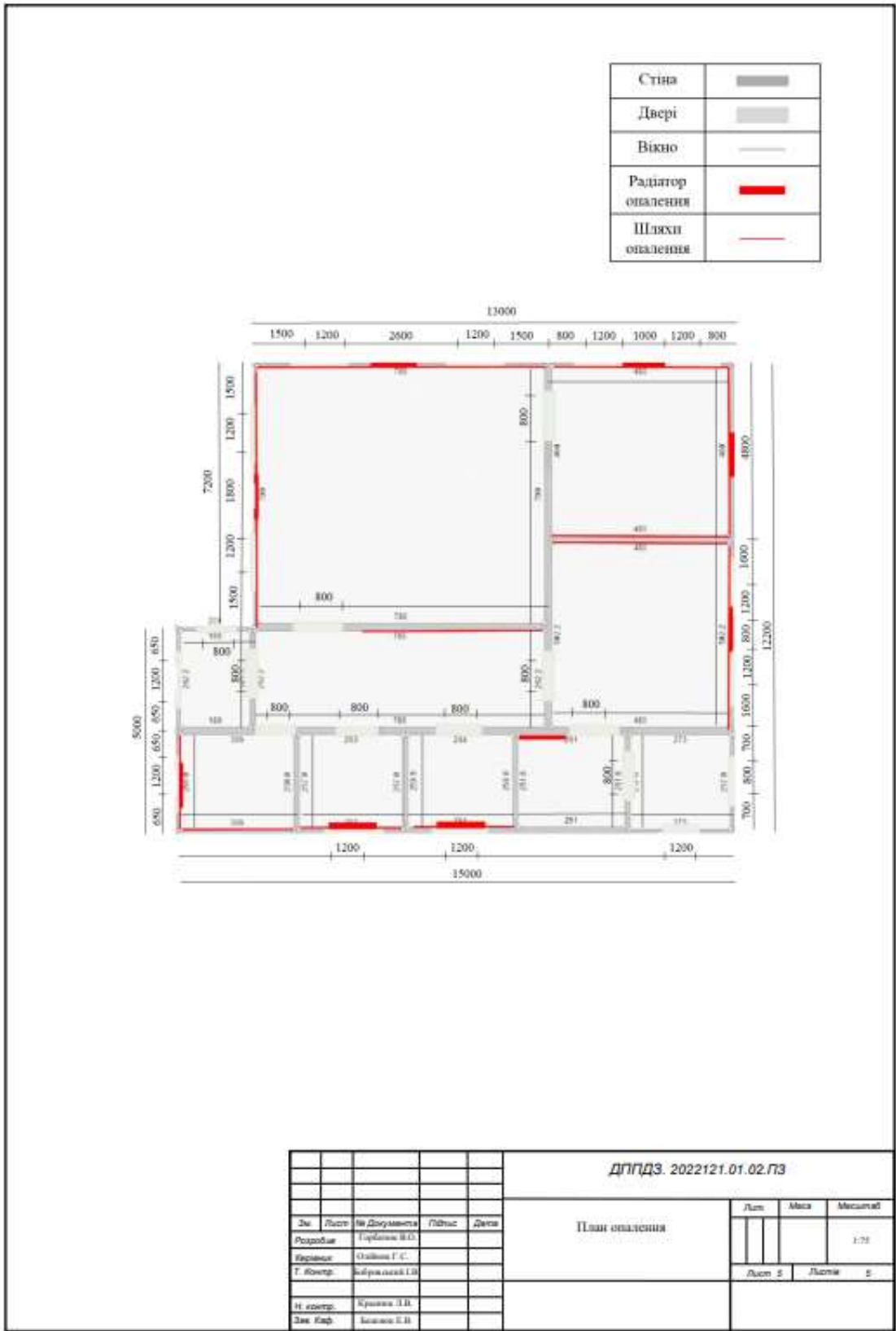
Рисунок А5 – План опалення
