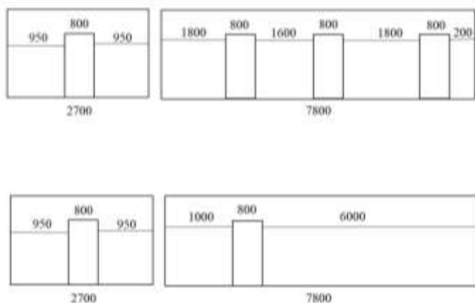
Рисунок 3.8 – Розгортки стін роздягальні
