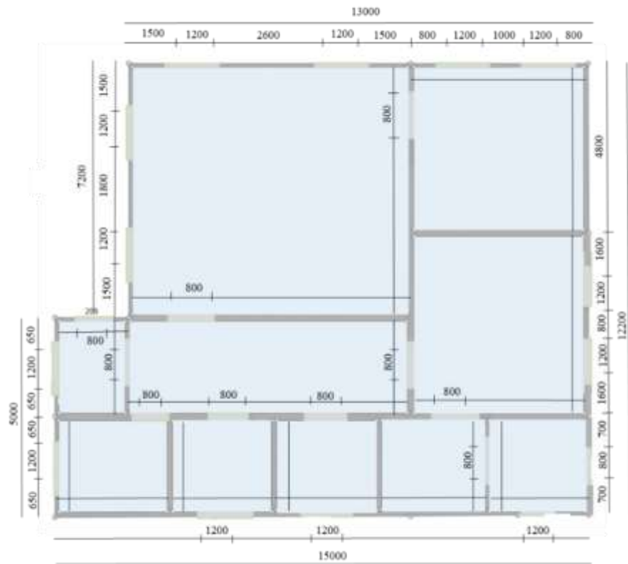
Рисунок 3.3 – План стелі
