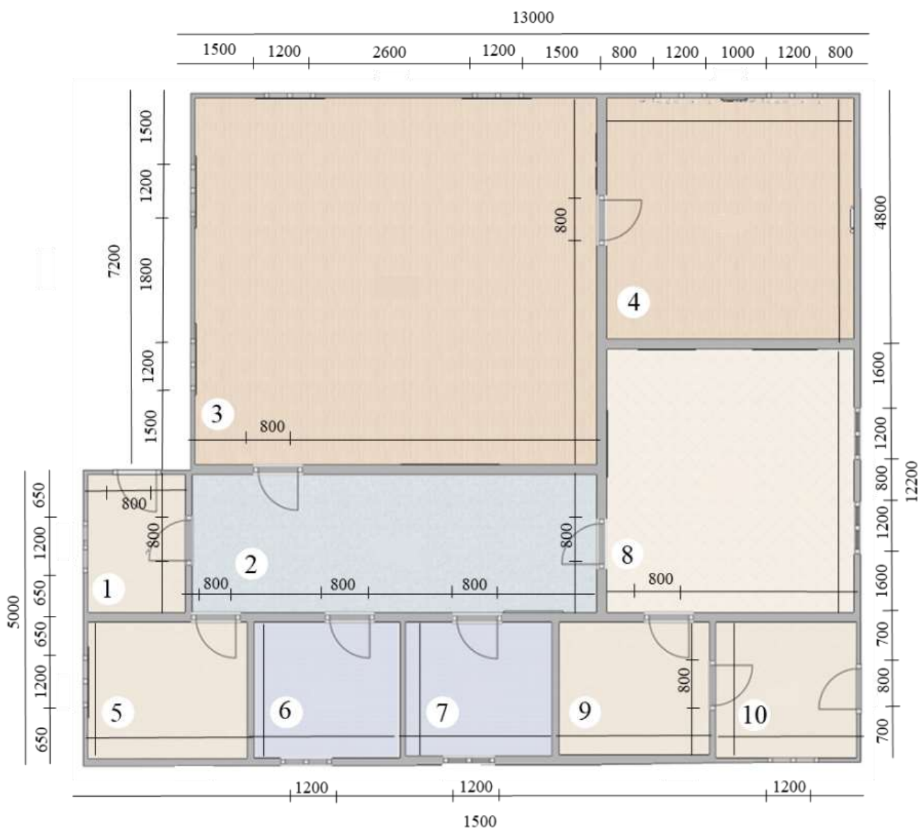
Рисунок 3.2 – План підлоги
