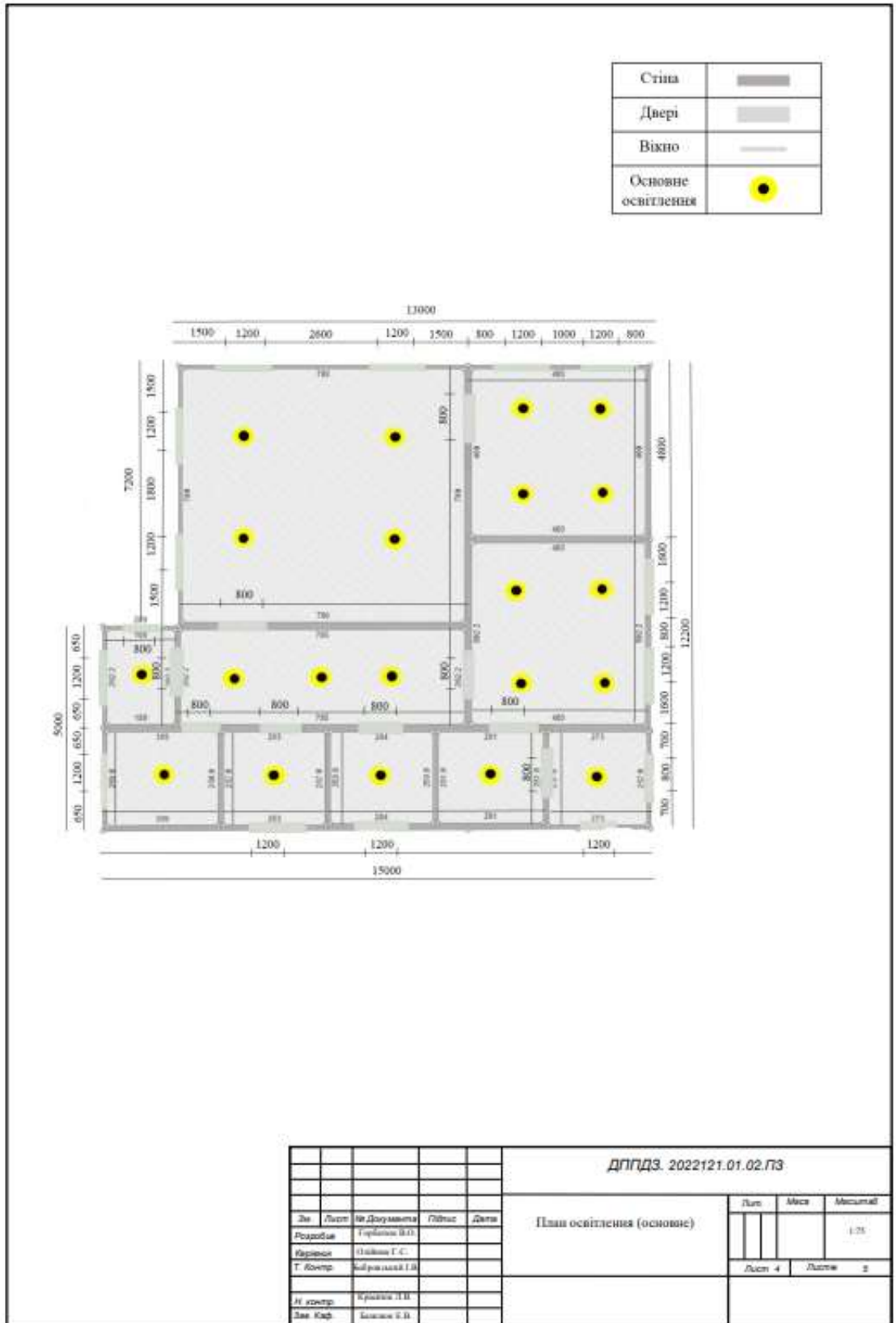
Рисунок А4 – План освітлення
