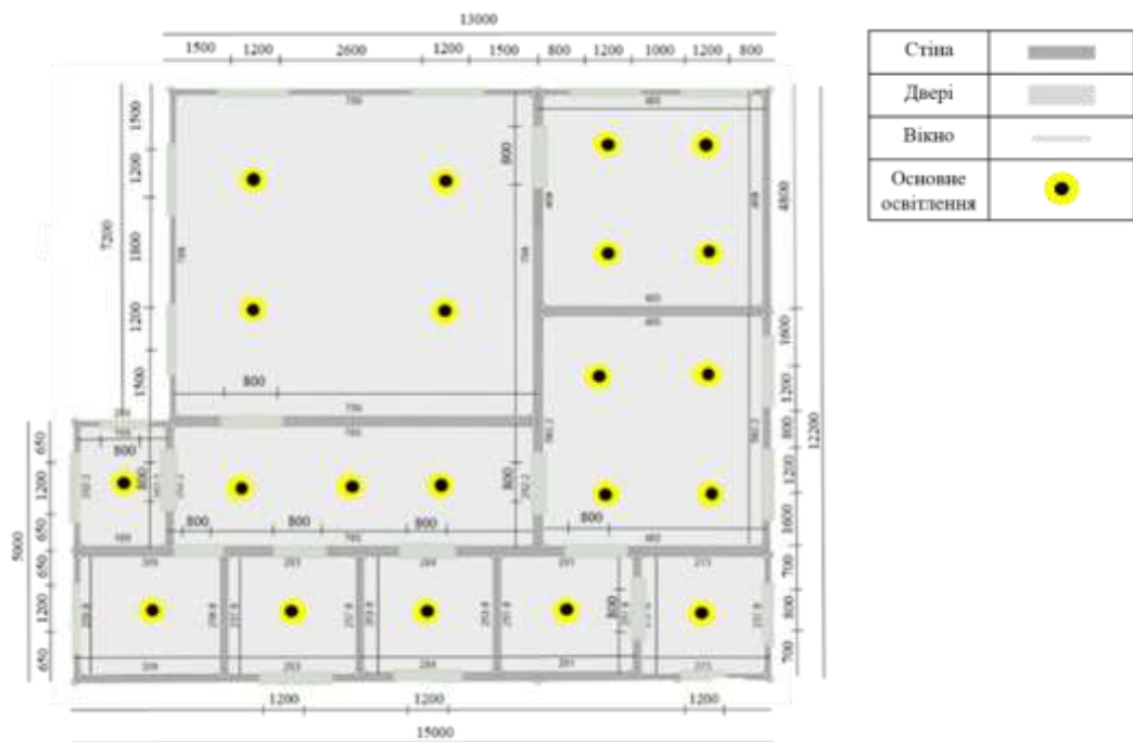
Рисунок 3.4 – План освітлення
