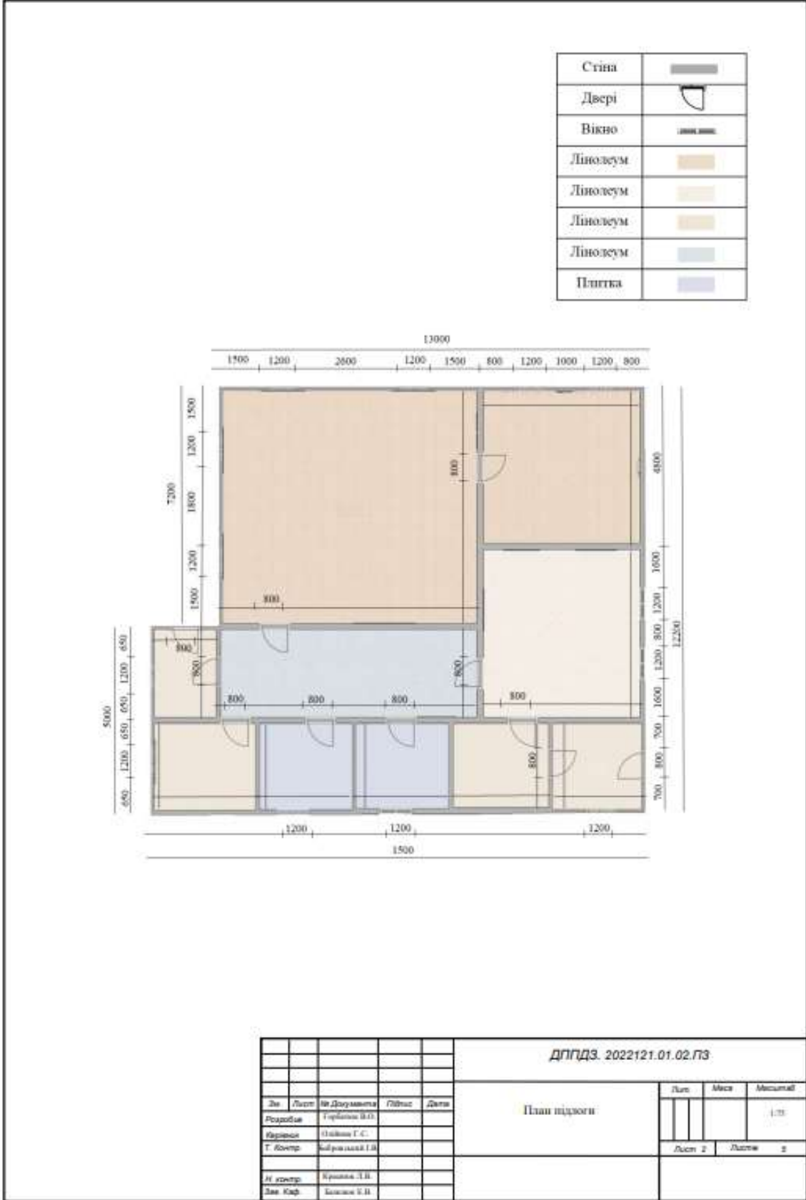
Рисунок А2 – План підлоги
