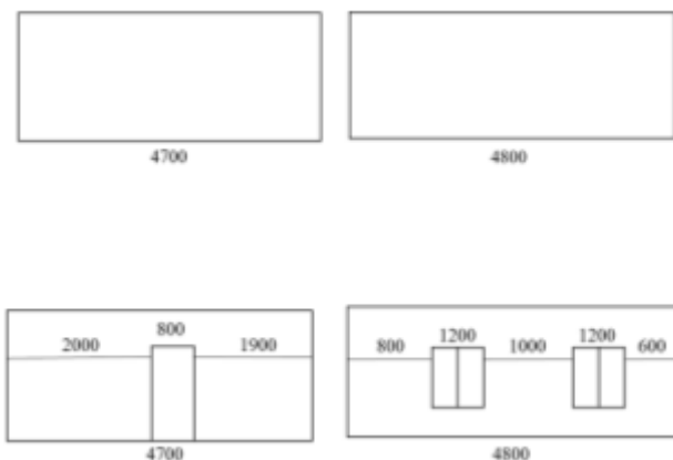
Рисунок 3.7 – Розгортки стін спальної кімнати
