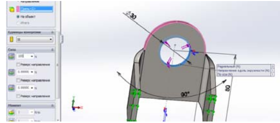
Рис. 3. Прикладання навантаження
