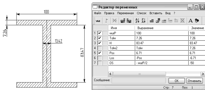
Рис. 10. Представлення у середовищі T-Flex
